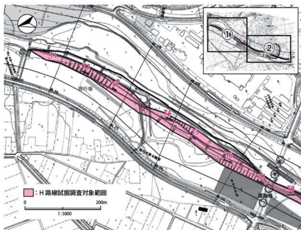
最上川上流河川改修事業（須川地区H路線①） トレンチ配置図
