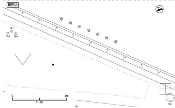
花ノ木遺跡 遺構配置図
