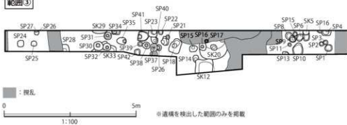
藤島城跡 遺構配置図
