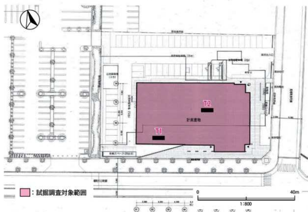
鶴岡第2地方合同庁舎建設 トレンチ配置図
