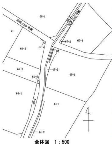
全体図 1:500
