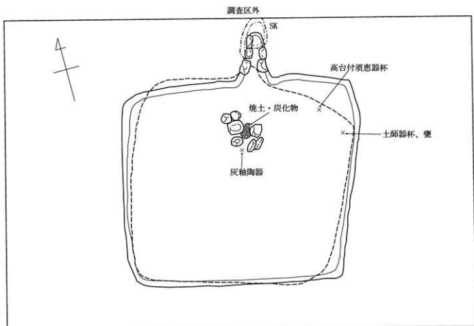
平面図 1 : 50
