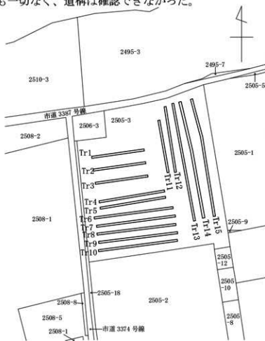
全体図 1:1,000
