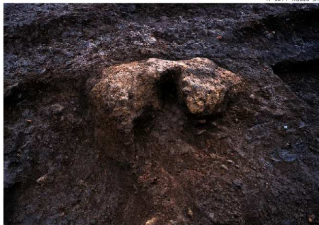
2. SB14 カマド (南西から)
