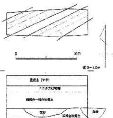
第52図 トレンチ4の平面図と土層断面図 (S=1/60)
