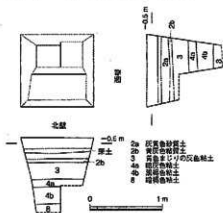
第21図 T-5 平面・断面図 (S=1/50)
