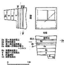
第31図 T-9 平面・断面図(S=1/50)
