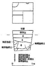
第13図 T-2平面・断面図(S=1/50)
