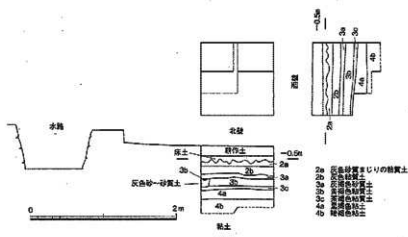
第9図 T-1 平面・断面図 (S=1/50)
