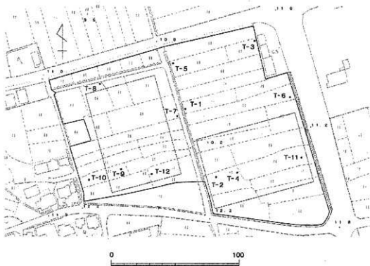
第8図 トレンチ配置図(S=1/2,000)
