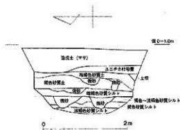
第51図 トレンチ3の平面図と土層断面図 (S=1/60)
