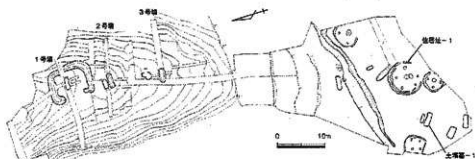
第60図 遺構配置図 (S=1/800)
