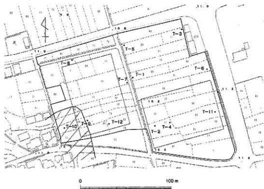
第40図 遺跡範囲図 (S=1/2,000)
