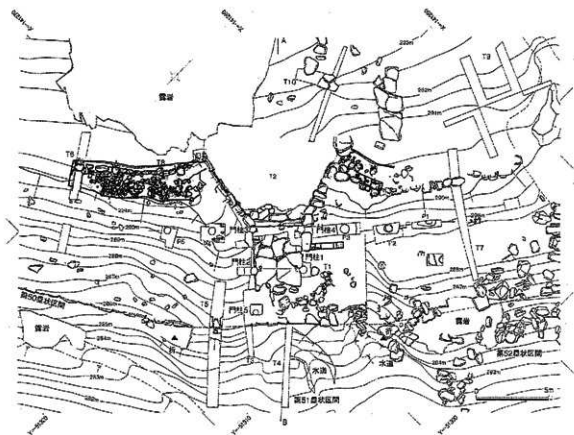
第 77 図 東門と内側列石と敷石の状況 (S = 1/200)
