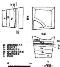
第37図 T-12 平面・断面図 (S=1/50)
