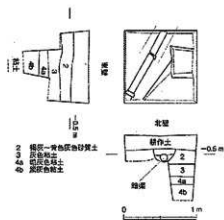
第28図 T-8 平面・断面図 (S=1/50)
