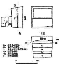
第35図 T-11 平面・断面図 (S=1/50)
