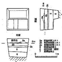
第17図 T-4 平面・断面図 (S=1/50)
