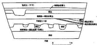
第44図 T-8土層断面 (S=1/60)
