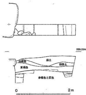
第73図 トレンチ 平・断面図 (S=1/40)
