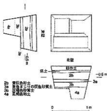
第23図 T-6 平面・断面図 (S=1/50)
