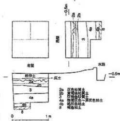
第16図 T-3 平面・断面図(S=1/50)
