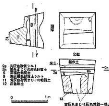
第34図 T-10 平面・断面図 (S=1/50)
