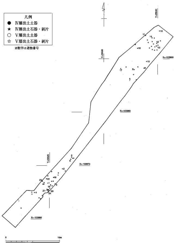
第10図 IV層・V層出土遺物分布図 (1/200)
