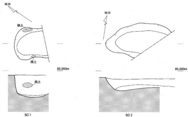
第8図 土坑実測図 (1/20)
