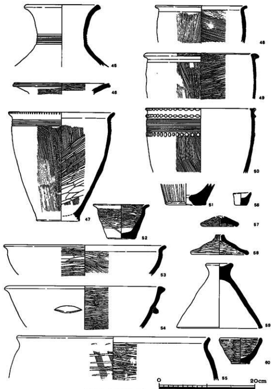
第9图 土器实测图V SD001上層
