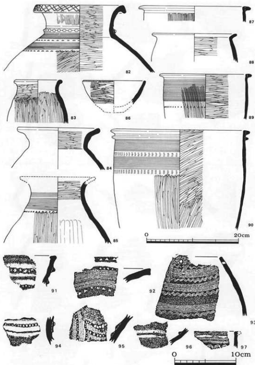
第11圖 土器実測図Ⅶ SD002
