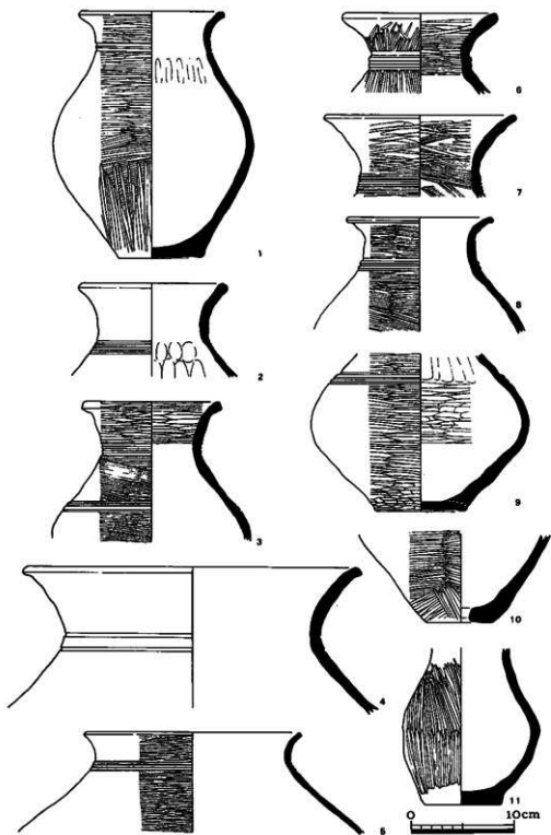
第5圖 土器実測圖 I SD001下層(5は \frac{1}{2} )
