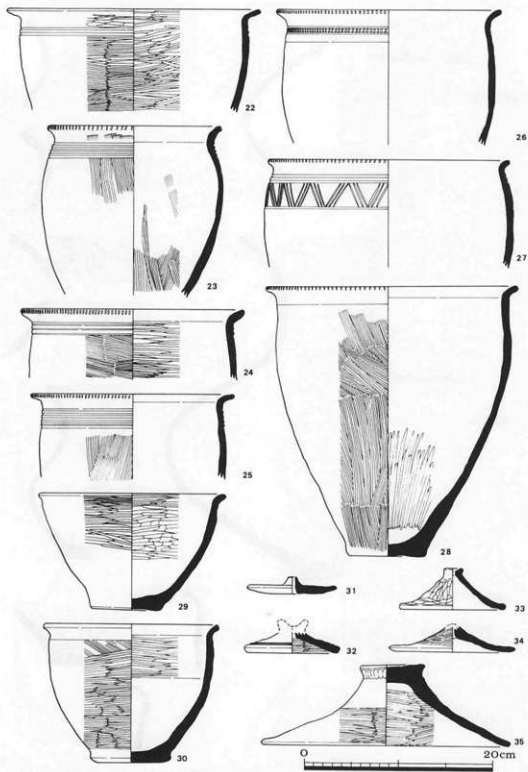
第7圖 土器実測圖Ⅲ SD001下層
