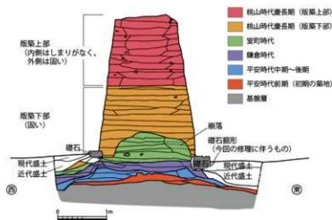
築地断面模式図
