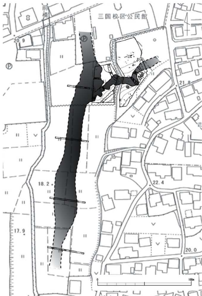
第7図 流路跡推定図 (S=1/1,250)
