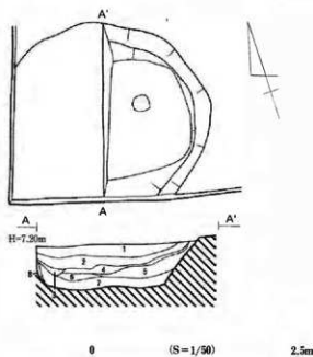
図13 18トレンチ平面図
