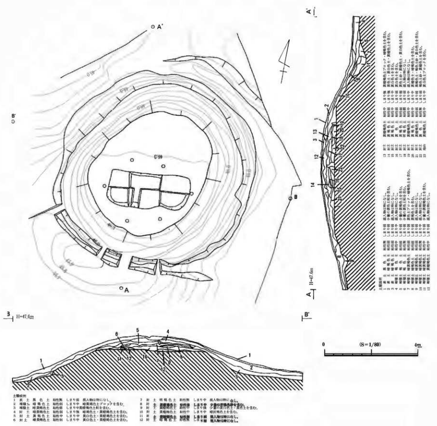
図3 1号墳平面図・断面図
