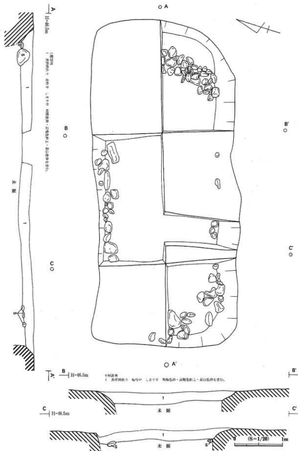
図4 埋葬施設平面図・断面図
