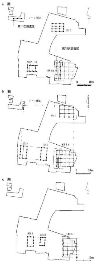
図17 建物群変遷図
