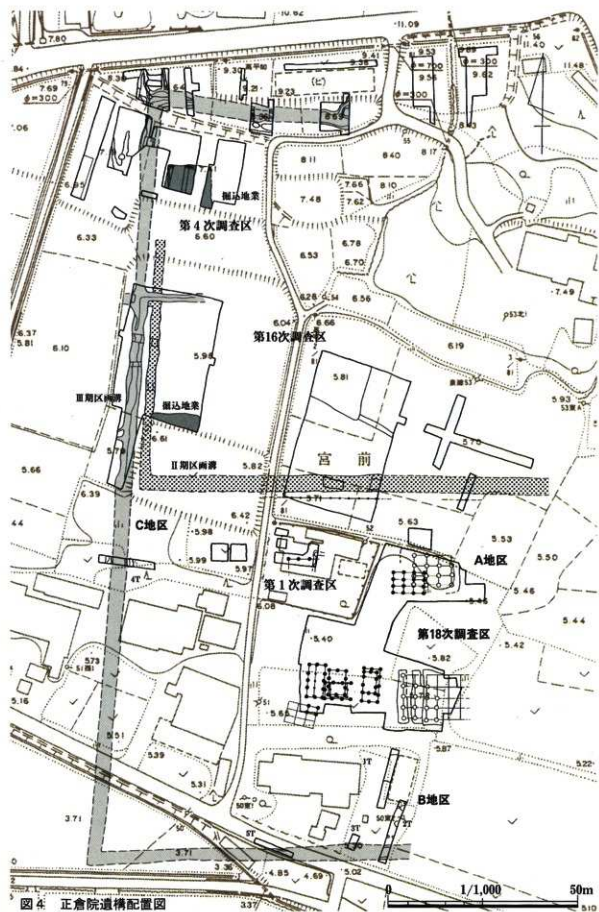
図4 正倉院遺構配置図
