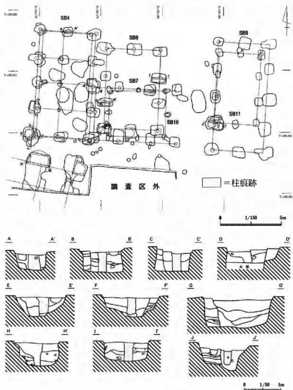
図9 A地区南西部掘立柱建物群
