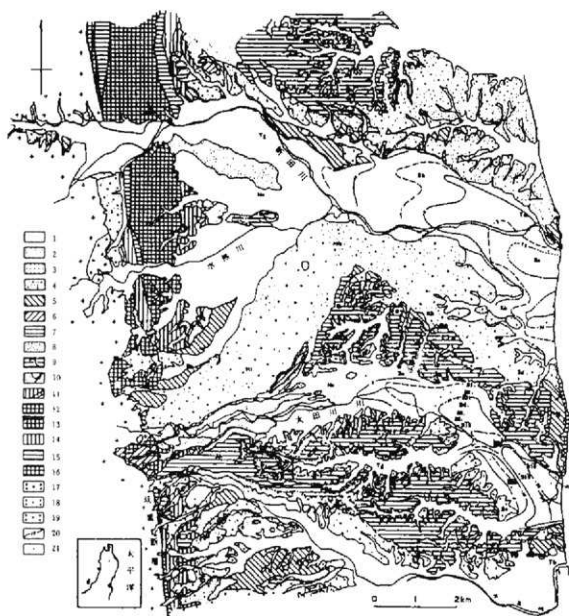
1: “沖積層”、2:第6段丘構成層、3:第5段丘構成層、4:第4段丘構成層、 5:第3段丘構成層、6:第2段丘構成層、7:第1段丘構成層、8~11:竜の 口層、8:同c層(砂岩)、9:同c層(シルト岩・京塚沢凝灰岩)、10:同b層、 11:同a層、12~19:基盤岩類、12:塩手層、13:小山田層、14:富沢層、15: 中の沢層、16:橋窪層、17:古生層、18:花崗岩類、19:脈岩、20:竜の口層上 面標高(m)、21:ボーリング地点と孔番、Ah:畦原、Bh:馬場、Hh:雲雀ヶ原、 Ith:原町市街、Ht:東高松、Ka:菅浜、Kh:北原、Kk:片倉、Mg:岡形沢、 Mn:米ヶ沢、Nn:長野、No:中太田、Om:大奥、Sd:幸、Se:下江井、Sk:下北 高平、So:下太田、Ss:F沢佐、Tb:塚原、Tg:鶴谷、Tn:船前、Yg:横上。
