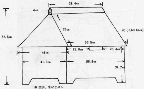
平面図② 素焼寄轆式厨子
