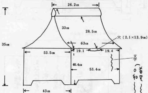
平面図⑥ 石灰岩製寄棟式厨子
