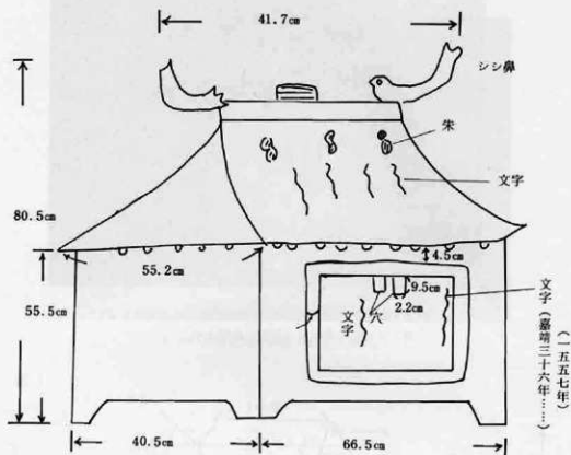
平面図② 石灰岩製寄棟式厨子
