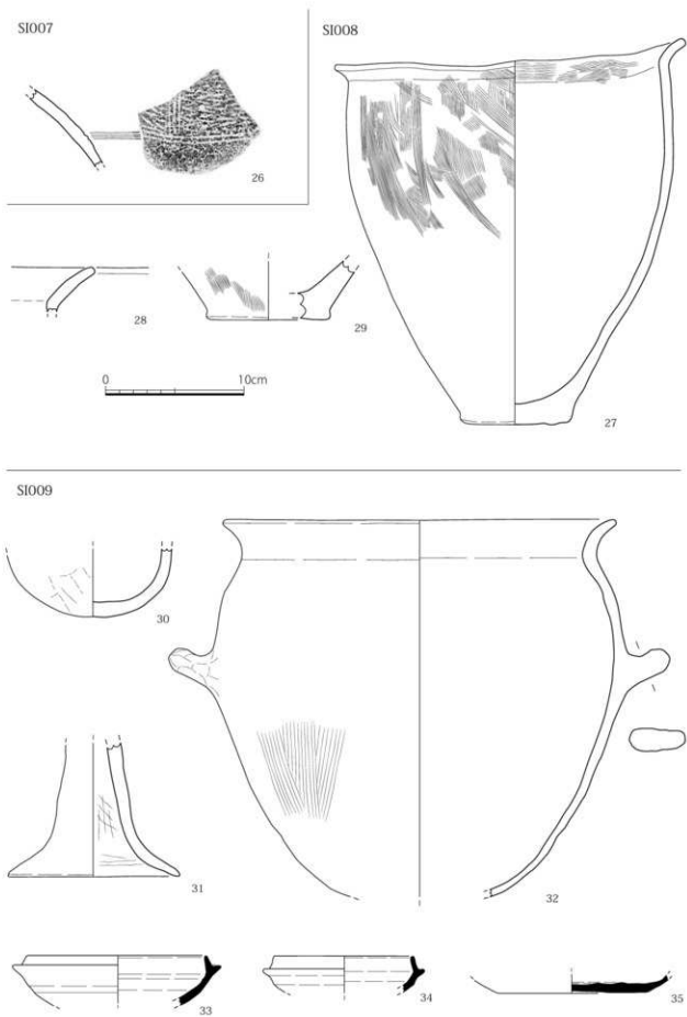
第15图 I区出土土器实测图5 (1/3)
