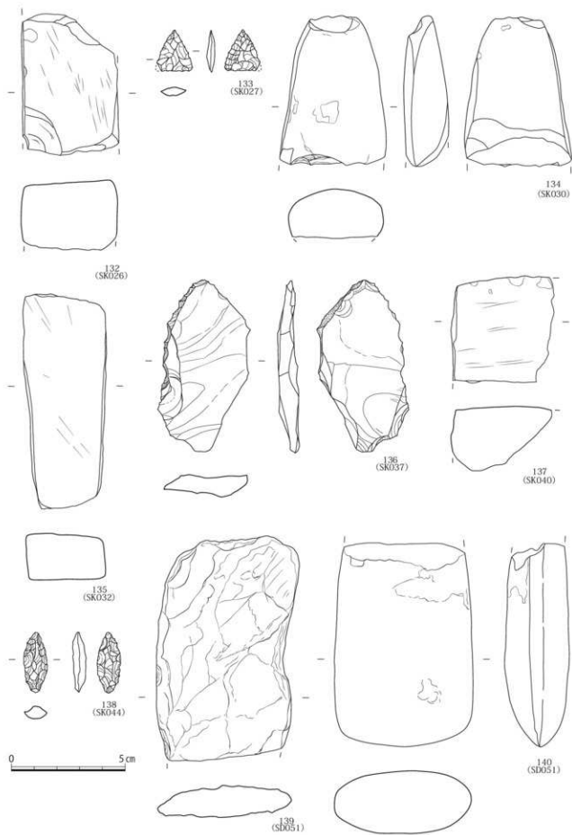
第 33 图 I 区出土石器实测图 4 (2/3)
