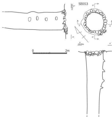
第28図 I区 SE053実測図 (1/60)
