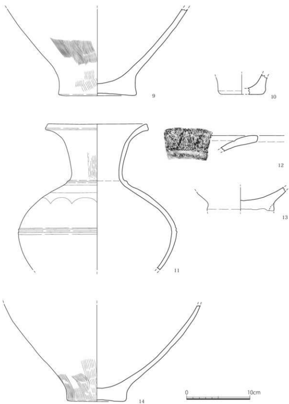
第10图 I区出土土器实测图3 (1/3)
