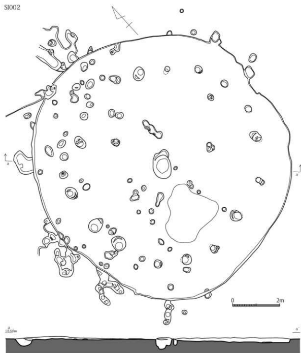
第8図 I区SI002実測図(1/80)
