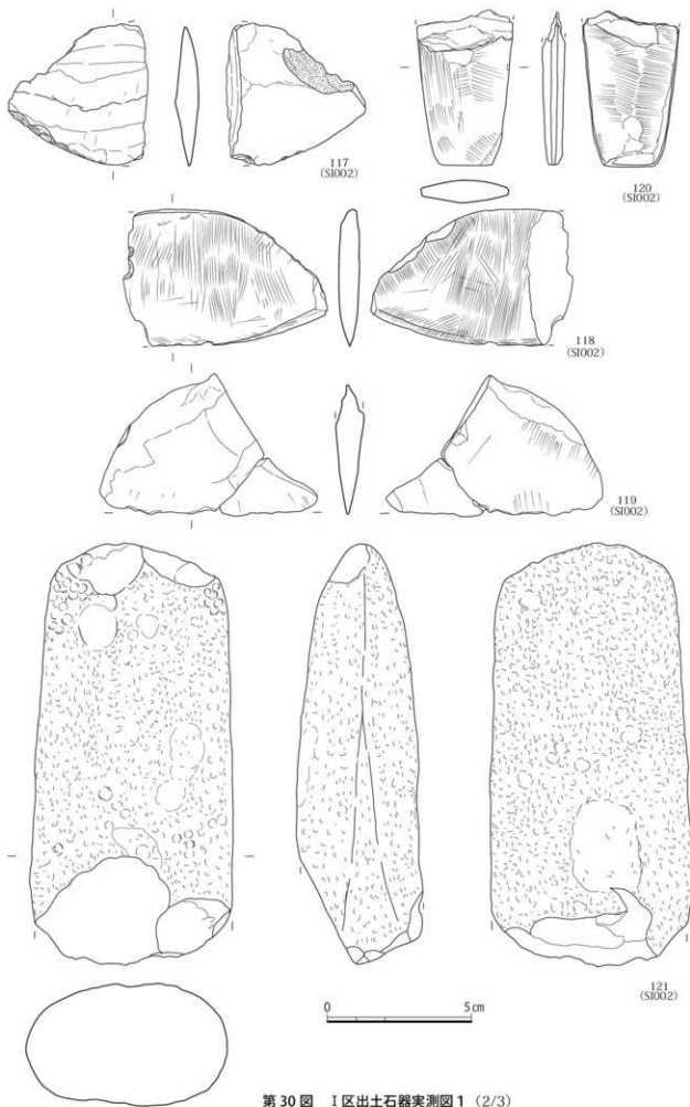
第30图 I区出土石器实测图1 (2/3)
