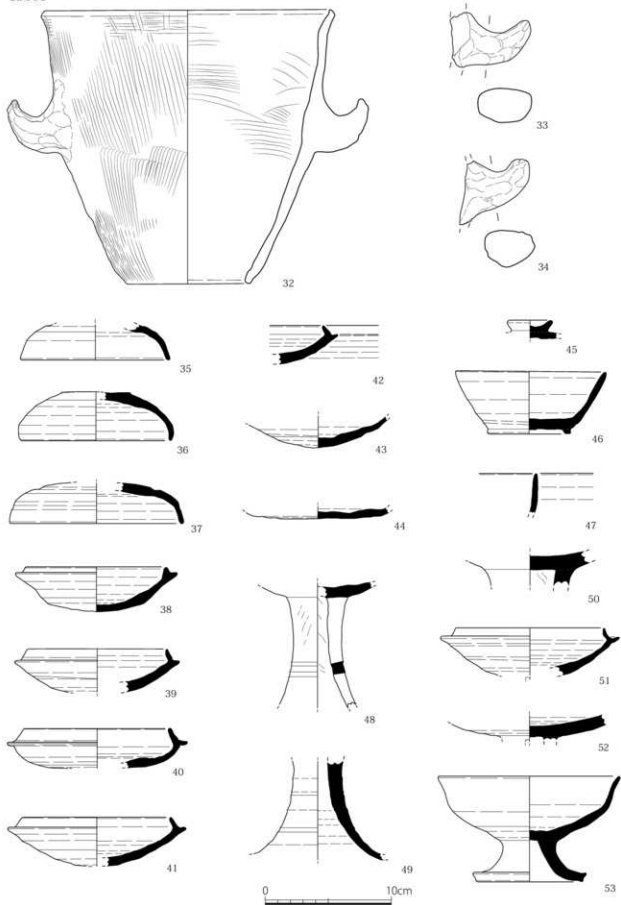
第42图 II区出土土器实测图4 (1/3)
