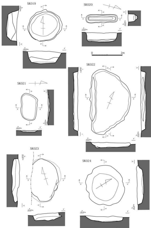
第 19 图 I 区 SK019 · 020 · 021 · 022 · 023 · 024 实测图 (1/60)
