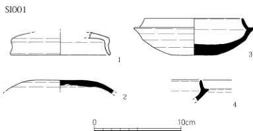
第7図 I区出土土器実測図1(1/3)
