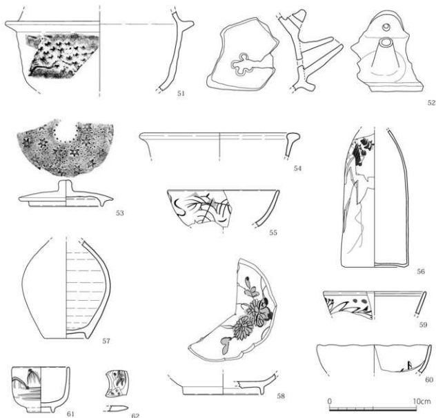
第21図 I区出土土器実測図7 (1/3)
