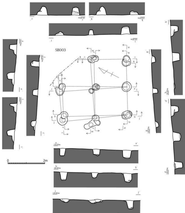
第38图 Ⅱ区SB003实测图(1/60)
