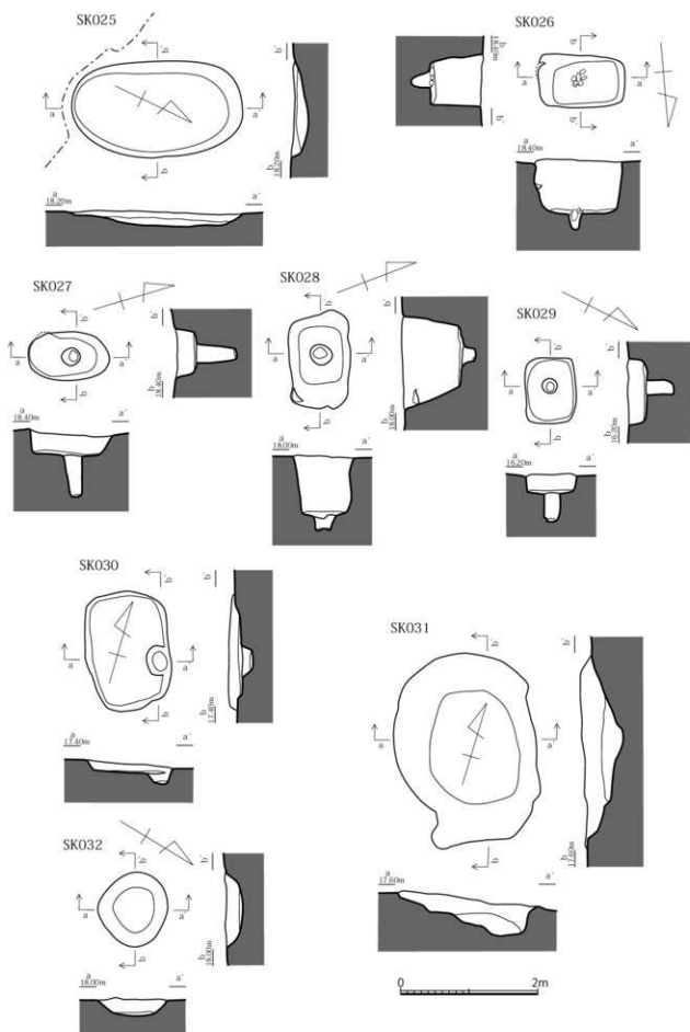
第20图 I区SK025·026·027·028·029·030·031·032实测图(1/60)
