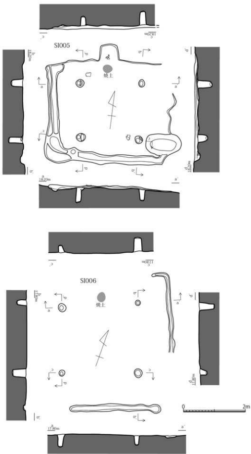
第 13 图 I 区 SI005 · 006 实测图 (1/60)
