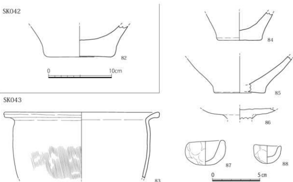
第25図 I区出土土器実測図10 (1/3・1/2)
