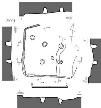
第6図 I区SI001実測図(1/60)
