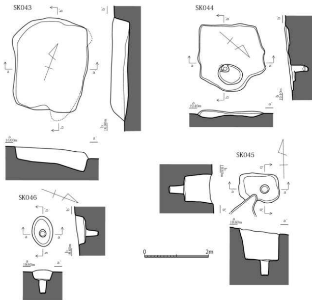
第26図 I区 SK043・044・045・046実測図 (1/60)
