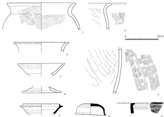
第37図 II区出土土器実測図1 (1/3)
