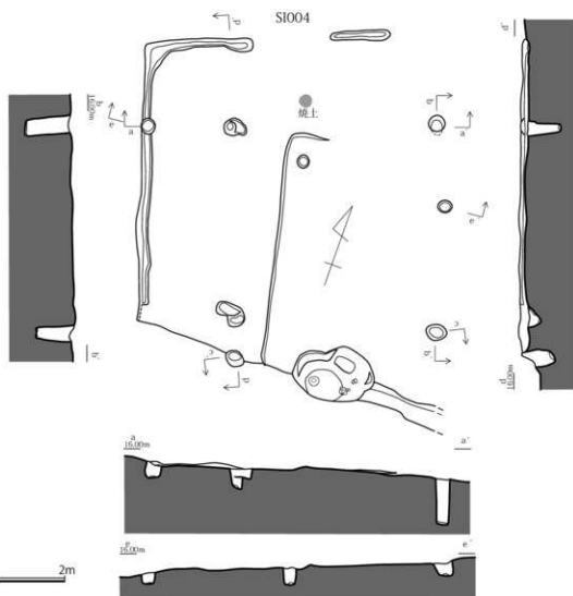
第11図 I区SI003・004実測図(1/60)
