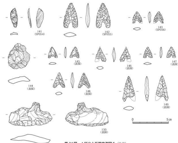
第34図 Ⅰ区出土石器実測図5 (2/3)
