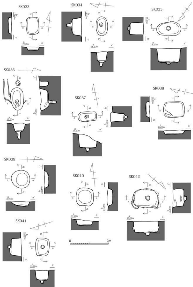
第 23 图 I 区 SK033 · 034 · 035 · 036 · 037 · 038 · 039 · 040 · 041 · 042 实测图 (1/60)
