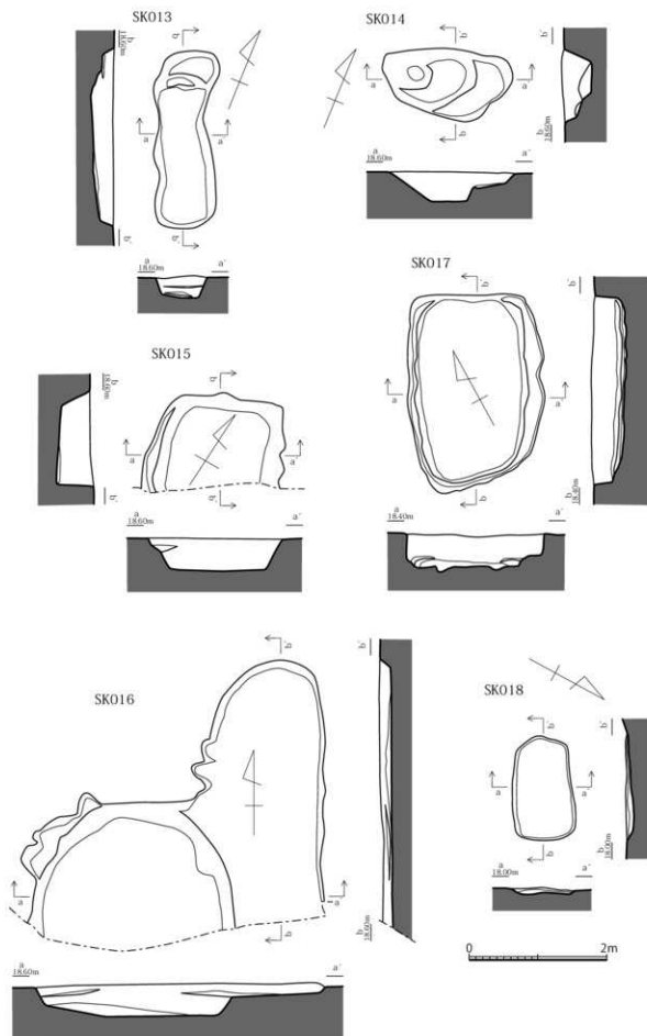
第 17 图 I 区 SK013 · 014 · 015 · 016 · 017 · 018 实测图 (1/60)
