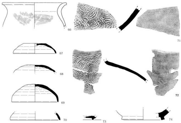
第 44 图 II 区出土土器实测图 6 (1/3)
