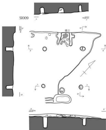
第14図 I区SI007・008・009実測図(1/60)
