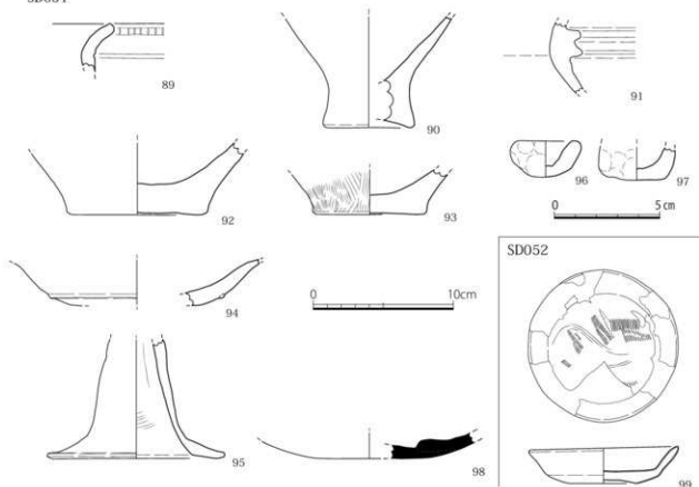
第27図 I区出土土器実測図11 (1/3・1/2)
