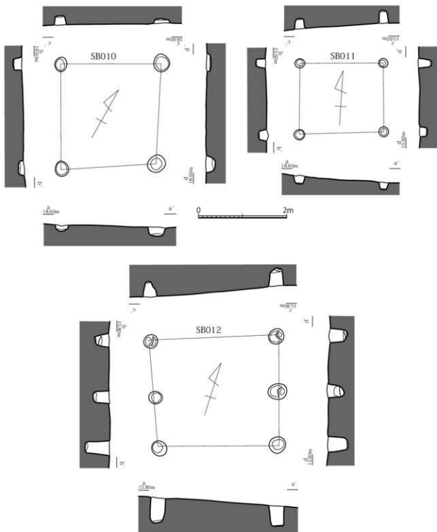
第16図 I区 SB010・011・012 実測図 (1/60)
