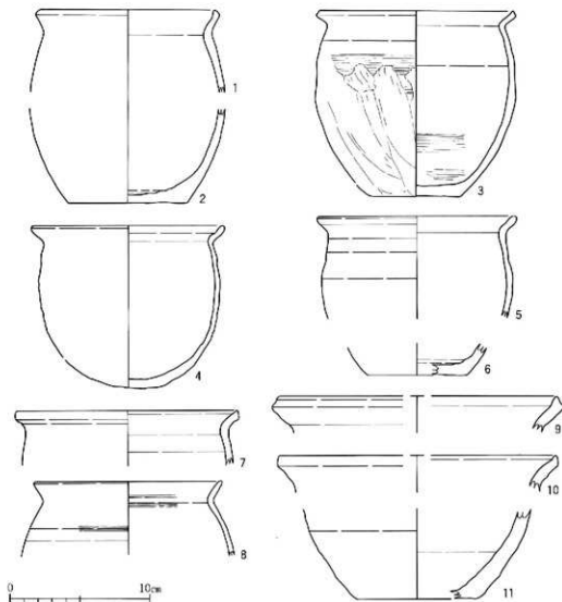
第9図 2T一括土器実測図(1/3)
