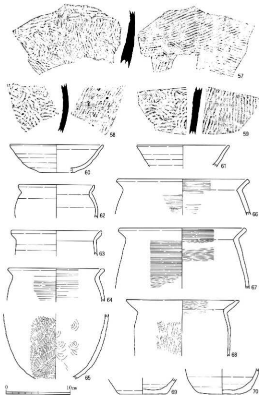
第12図 遺物実測図(1/3)
