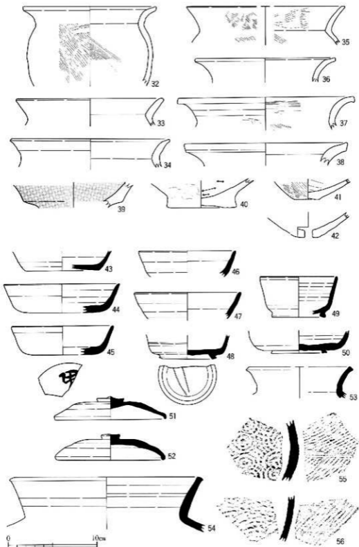
第11图 遺物実測図(1/3)
