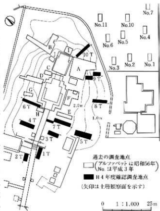
第5図 トレンチ設定図(1/1,000)
