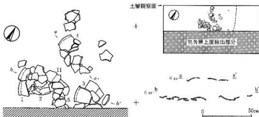
第8図 2T一括土器出土状況(1/20)
