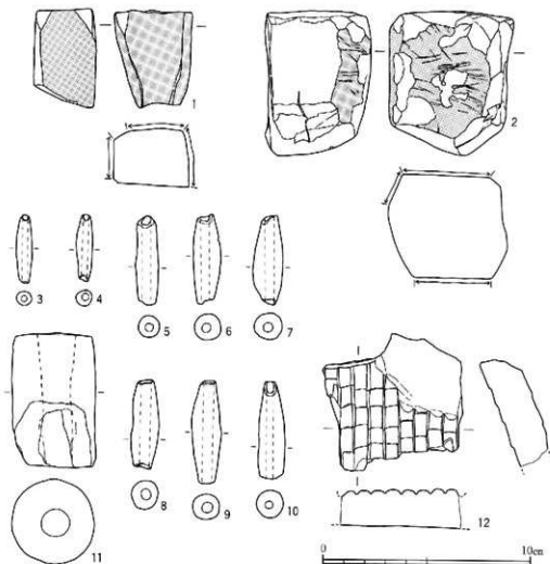
第13図 石製品・土製品実測図(1/2)
