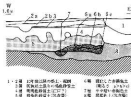
第7図 2T断面土層図(1/60)
