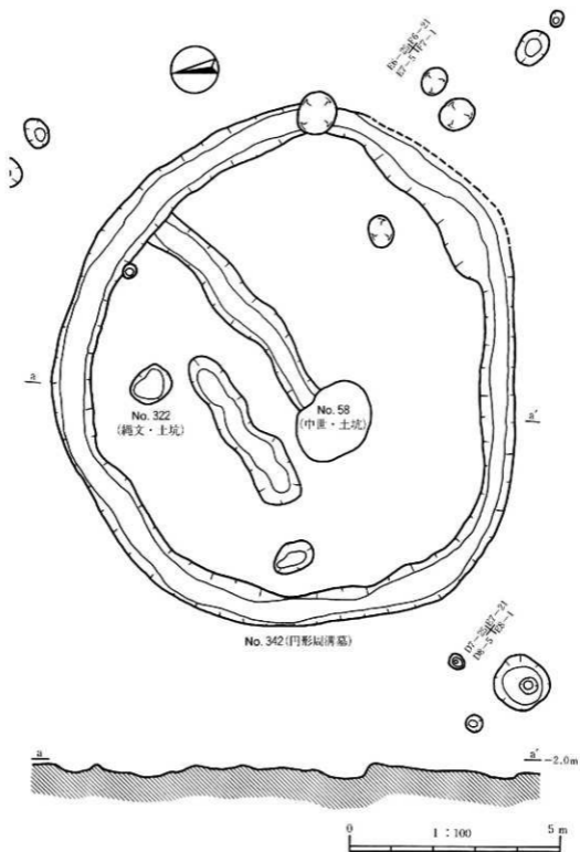
第13図 遺構実測図(第4回ブロック7)
