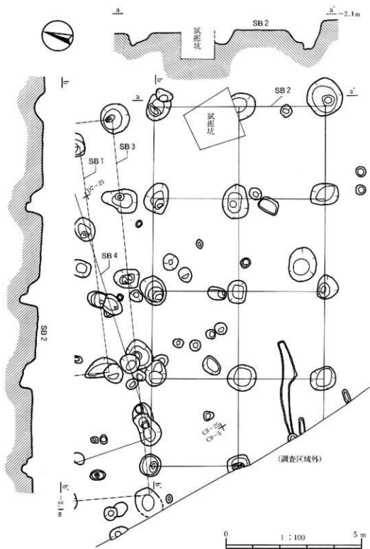
第12図 遺構実測図(第4回ブロック6)
