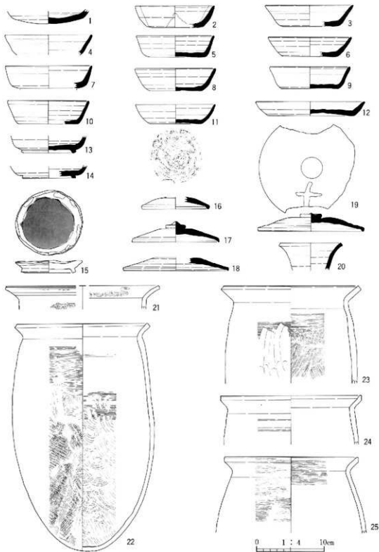
第14圖 遺物実測図(No. 440遺構)
