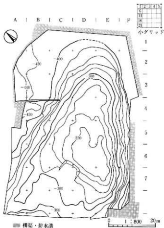
第3図 地形測量とグリッド設定図(1/800)
