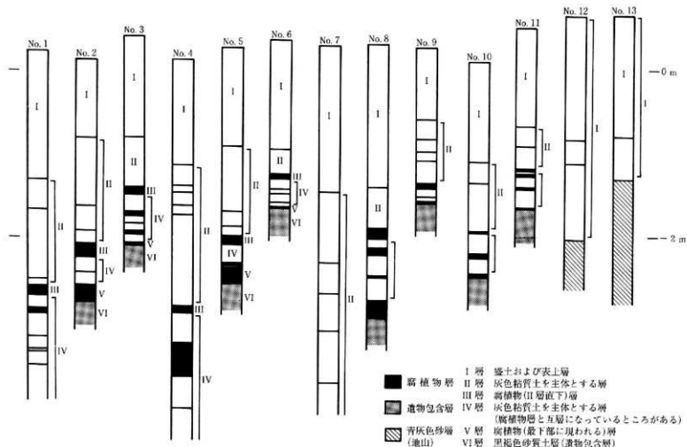
第3図 土層柱状図(1/40)
