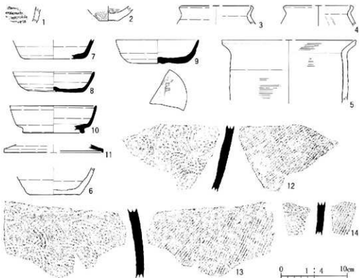
第4図 遺物実測図(1/4)
