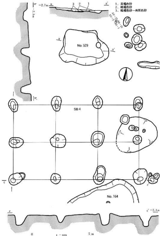
第8図 遺構実測図(第4図ブロック2)
