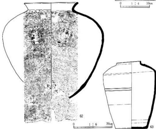
第16図 遺物実測図(土器破り1)
