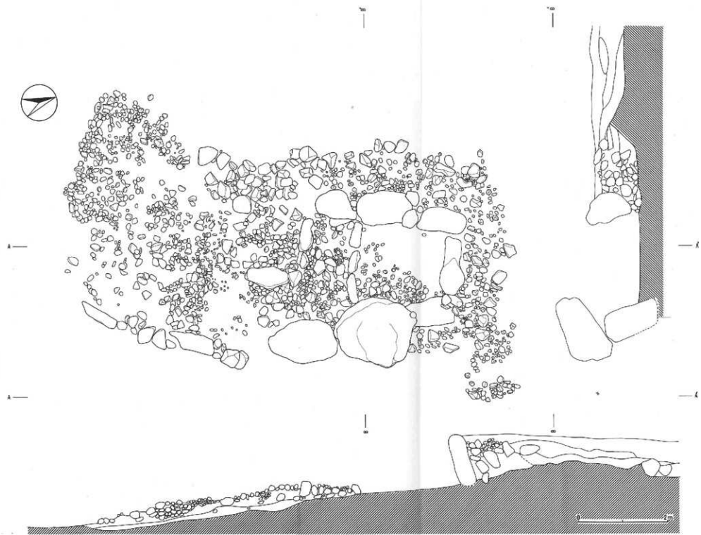
第4圖 下大豆塚1号古墳石室実測圖(1:60)
