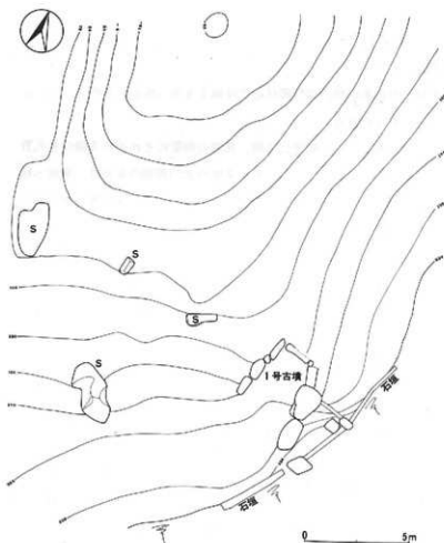
第3図 下大豆塚1号古墳地形図(1:200)
