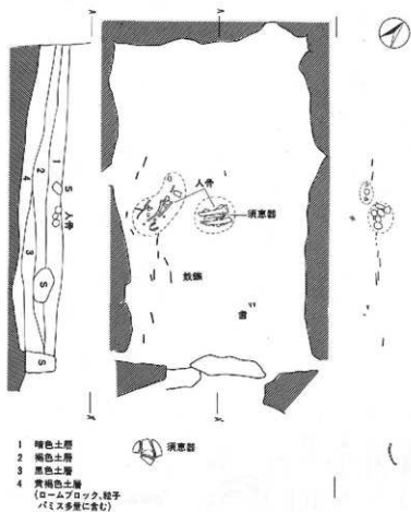
第11図 下大豆塚2号古墳石室内遺物分布図(1:30)
