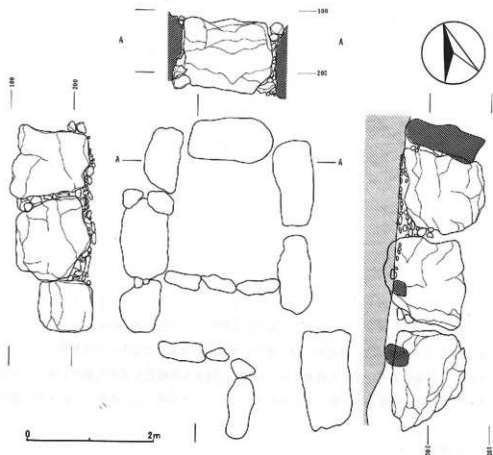
第5図 下大豆塚1号古墳石室展開図(1:60)
