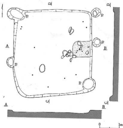
第47図 第19号住居址実測図 (H-19住) (1:60)
