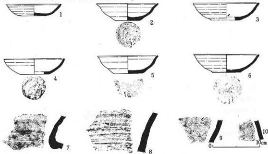
第33図 第12号住居址出土遺物実測図（1：4）
