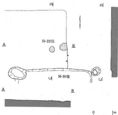
第55図 第22号住居実測図〔H-22住〕(1:60)
