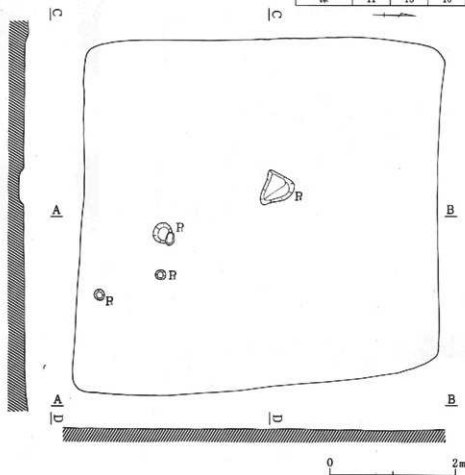
第11図 第4号住居址実測図〔H-4住〕(1:60)
