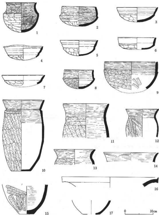
第9图 第1号住居址出土遗物实测图(1:4)
