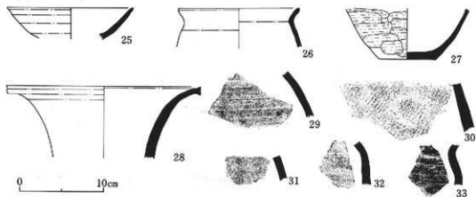
第46図 第18号住居址出土遺物実測図(1:4)
