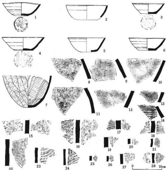
第13図 第2号住居址出土遺物実測図(1:4)
