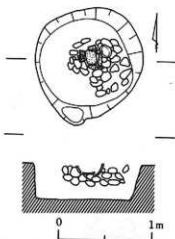
第4図 第1号土壇実測図 〔SK-01〕（1：60）
