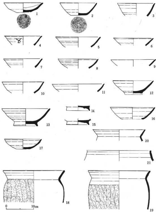
第48图 第19号住居址出土遺物実測図(1:4)
