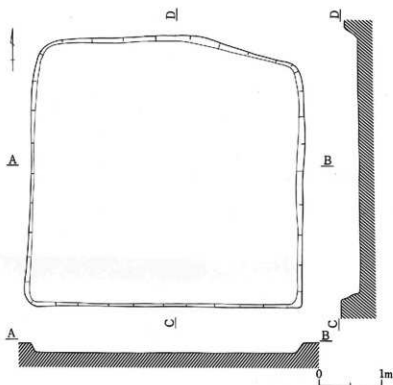
第58図 第24号住居址実測図〔H-24住〕（1：60）
