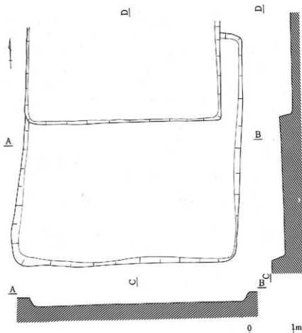
第59図 第25号住居址実測図〔H-25住〕(1:60)
