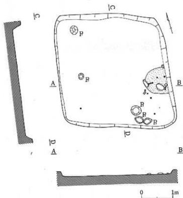
第19図 第6号住居址実測図（H-6住）（1:60）
