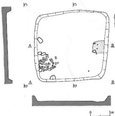
第21図 第7号住居址実測図(H-7住)(1:60)
