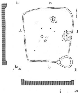
第44図 第18号住居址実測図〔H-18住〕(1:60)
