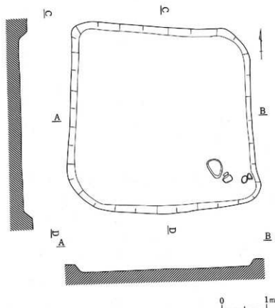
第61図 第27号住居址実測図〔H-27住〕(1:60)
