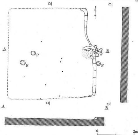
第25図 第9号住居址実測図〔H-9住〕(1:60)
