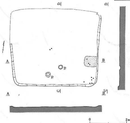
第29図 第11号住居址実測図〔H-11住〕(1:60)
