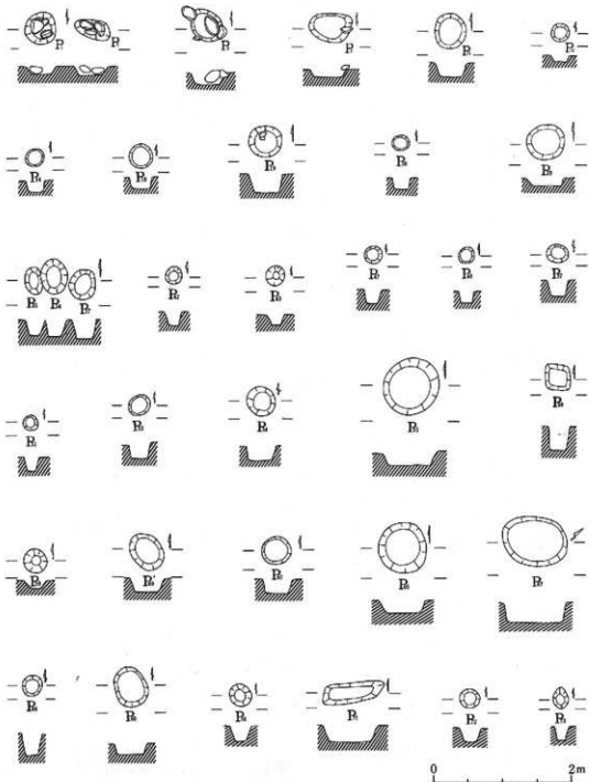
第66圖 第1・4・11~12・14・18~20・29・27・34・35・37・ 27・29 42・43・47・48・51・52・54・55・58~60・62・65・67 ~73号ピット実測図 (P: P 1 ...表示) (1:60)
