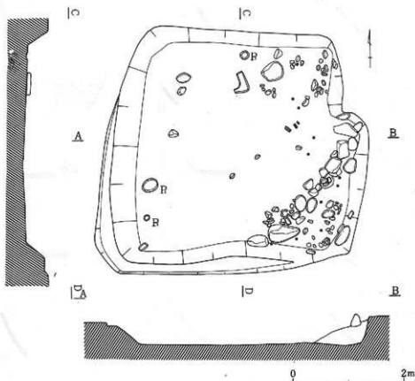
第14図 第3号住居址実測図 (H-3住) (1:60)
