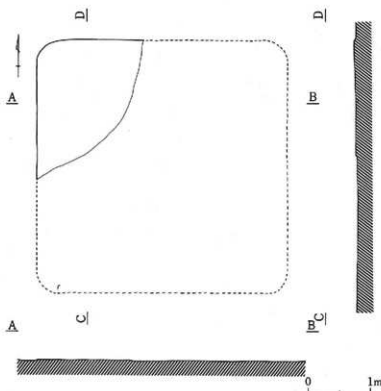
第57図 第23号住居址実測図〔H-23住〕（1：60）
