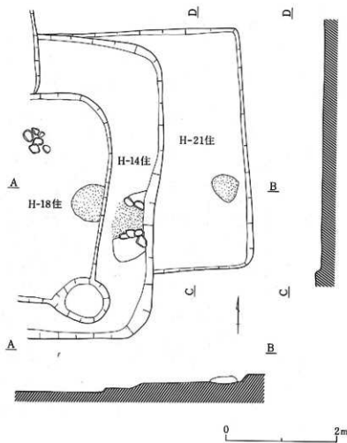
第53図 第21号住居址実測図〔H-21住〕(1:60)
