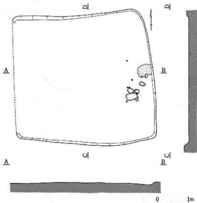
第32図 第12号住居址実測図〔H-12住〕（1：60）
