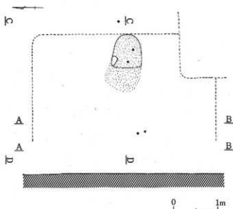
第27図 第10号住居址実測図〔H-10住〕（1：60）
