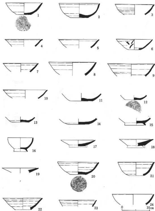
第45图 第18号住居址出土遗物实测图(1:4)
