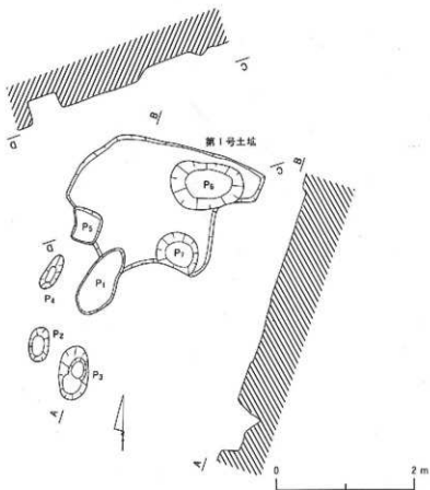
第6図 第1号土壇(SK-01)及びピット群実測図(1:60)
