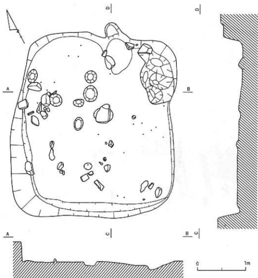
第3図 第1号住居址実測図 (1:40)
