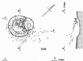
図面23 421次調査 SS57・59・60集石実測図
