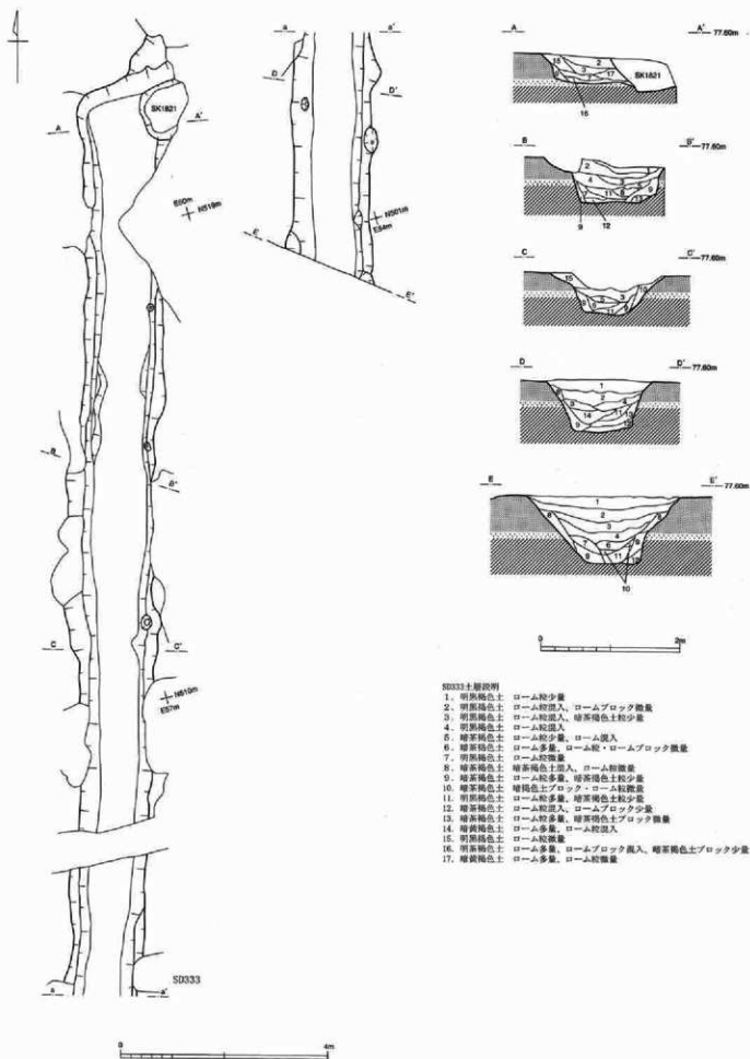
図面142 442次調査 SD333溝実測図
