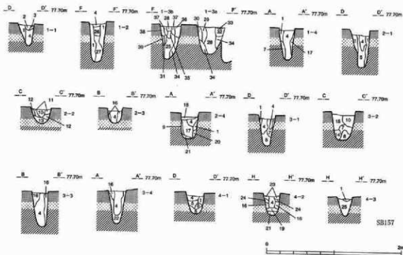
図面48 431・460次調査 SB157・160獨立柱建物実測図
