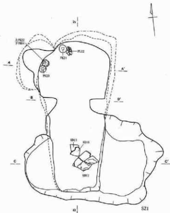
図面14 421次調査 SZ1 地下式横穴墓実測図
