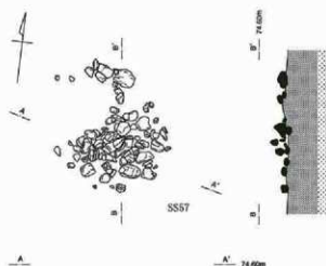
図面23 421次調査 SS57・59・60集石実測図
