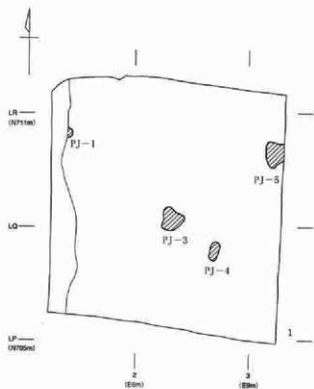
図面30 421次調査 SS57集石、SK1576J・1577J土坑、PJ-1～5・7～9 実測図
