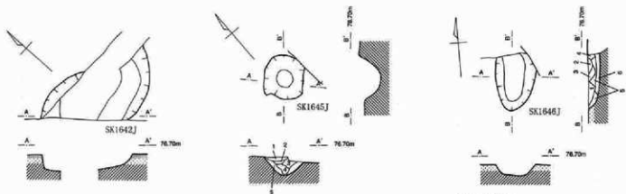
図面28 421次調査 SK1641J~1646J・1812J土坑実測図
