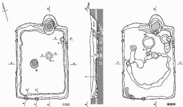
図面73 431次調査 SI552住居実測図
