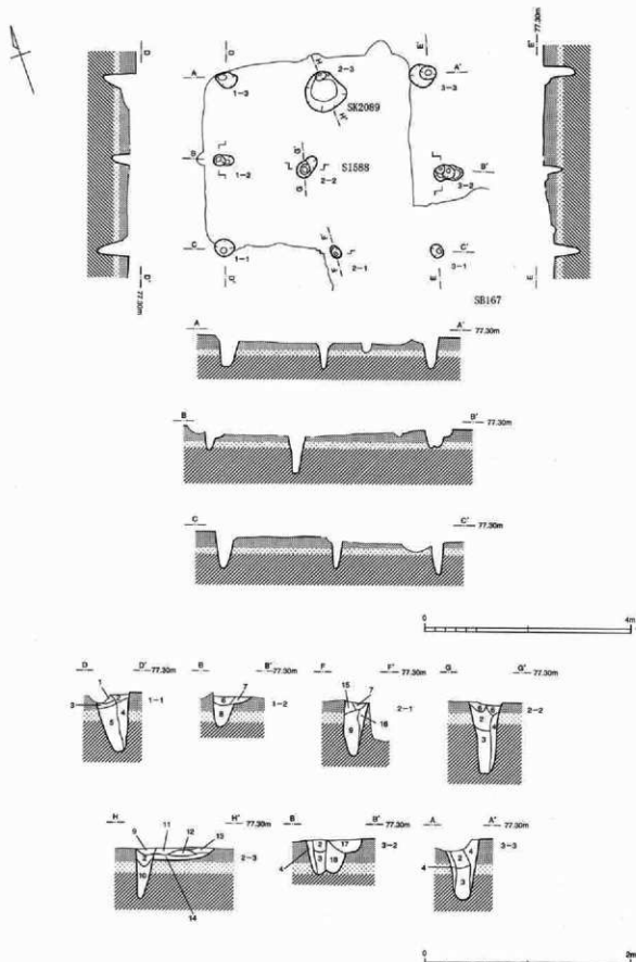
図面56 460次調査 SB167獨立柱建物実測図
