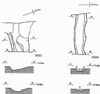
図面10 421次調査 SD318・321~323溝実測図
