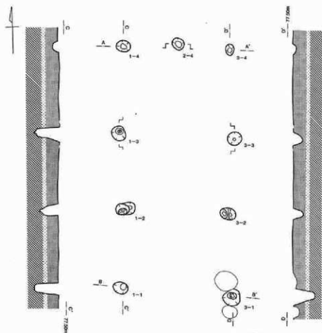
図面53 460次調査 SB164掘立柱建物実測図
