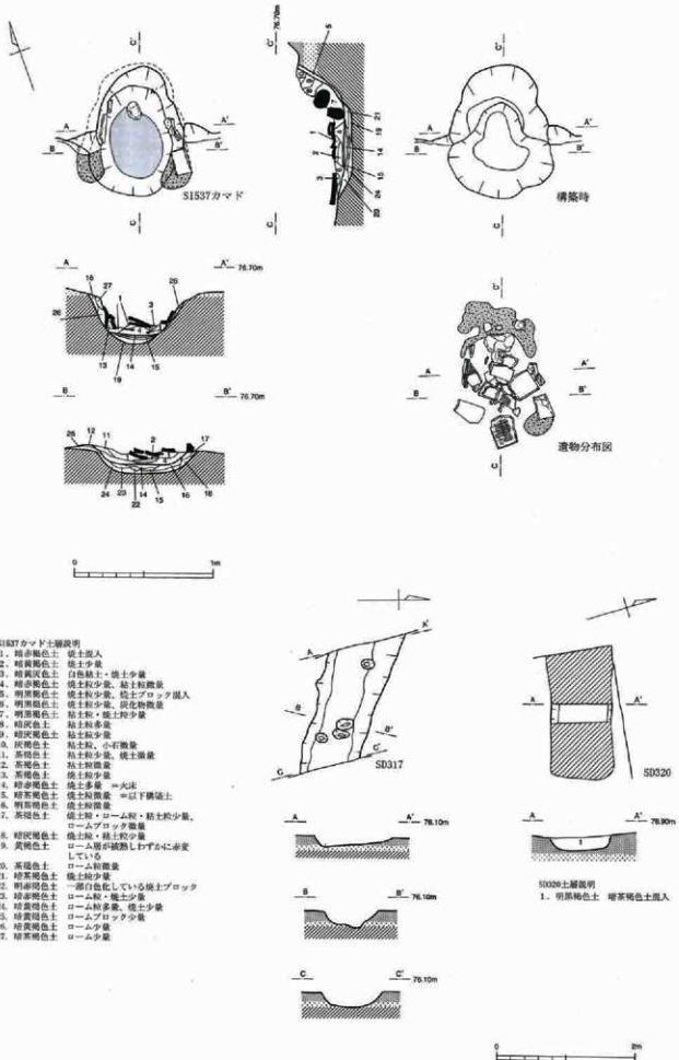
図面 8 421次調査 SI537住居カマド、SD317-323溝実測図
