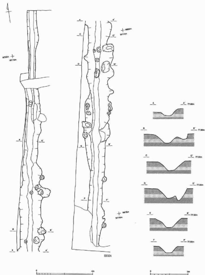
図面38 428次調査 SD324清実測図
