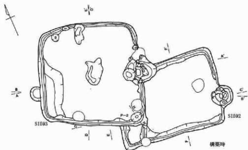
図面89 460次調査 S1592・593住居実測図
