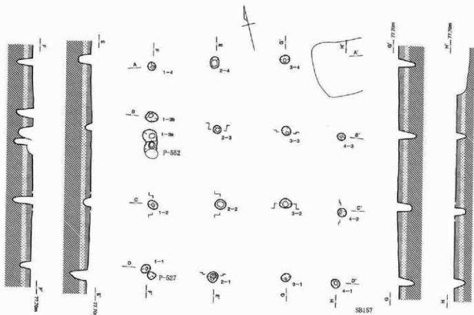
図面47 431次調査 SB157掘立柱建物実測図
