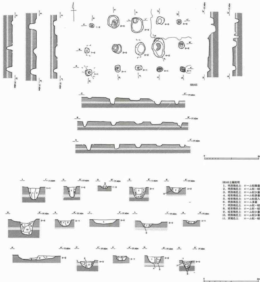
図面54 460次調査 SBI65竪立柱建物実測図
