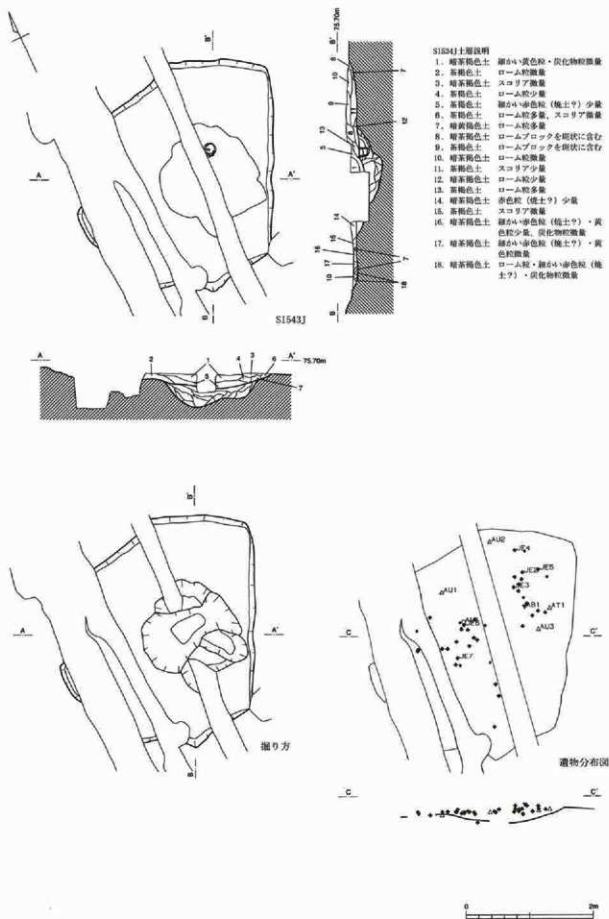
図面21 421次調査 SI543J住居実測図
