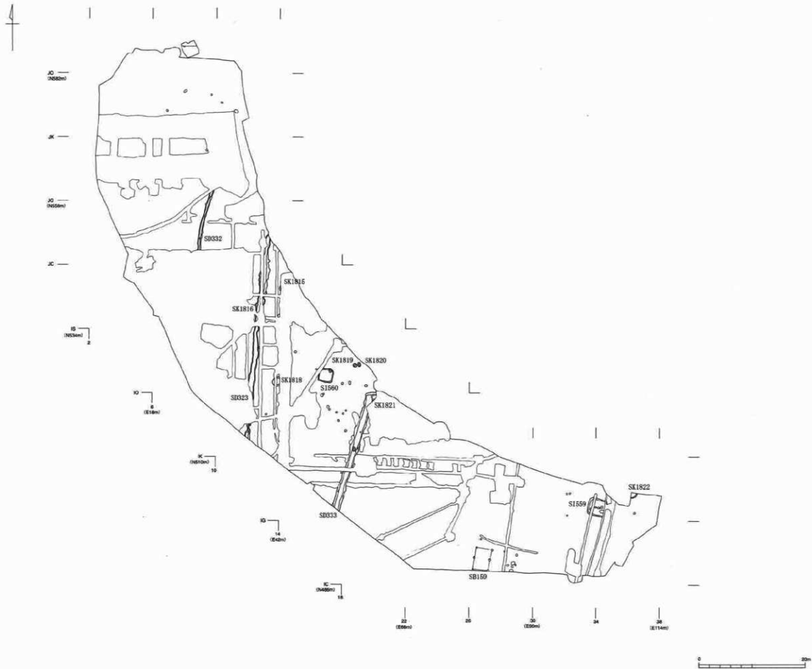
図面136 442次調査 歴史時代遺構配置図
