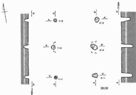
図面137 442次調査 SB159掘立柱建物実測図
