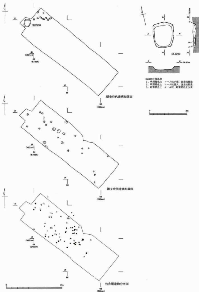
図面182 449次調査 歴史・縄文時代遺構配置図、包含層出土遺物分布図、SK1900土坑実測図
