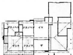
↓長野県三家復元平面図 1/300
