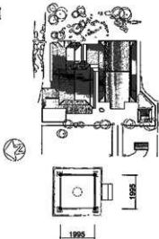
↑ 明秀寺鐘楼平面図 1/200
