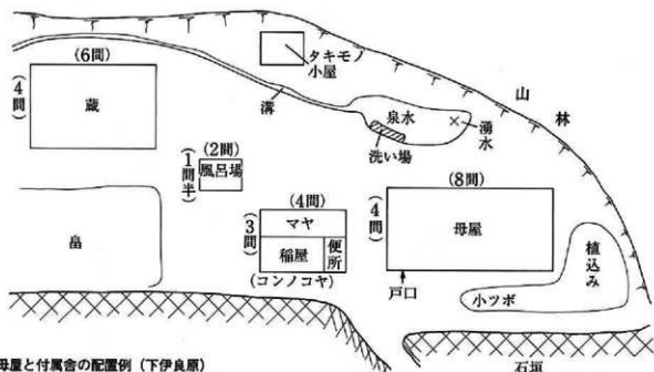
3 母屋と付属舎の配置例 (下伊良原)
