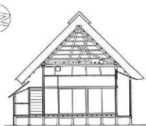
↑ 白川亘家断面図 1/200
