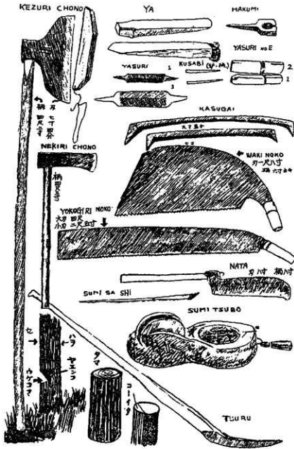
図3 山仕事道具
