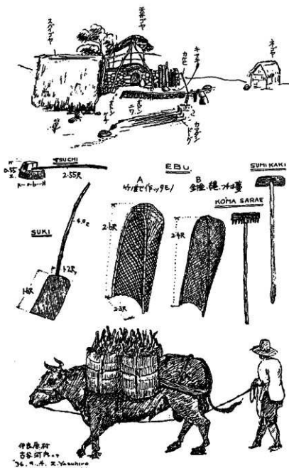
図4 炭焼用具
