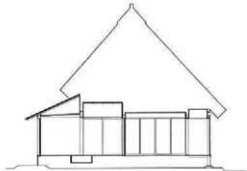
↑ 谷マサ子家復元平面図 1/300 ← 谷マサ子家断面図 1/200
