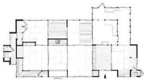
↑ 白川照子家現況平面図 1/300
