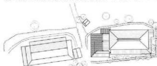
↑ 緒方寅夫家配置図 1/500
