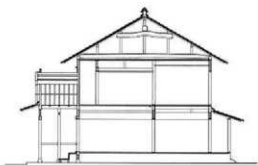
↑進時彦家断面図 1/200
