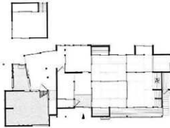
↑ 緒方寅夫家現況平面図 1/300
