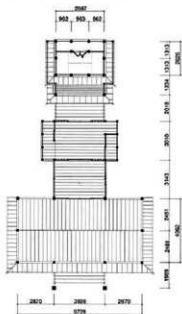
↑高木神社 (下) 神殿・拝殿平面図 1/300
