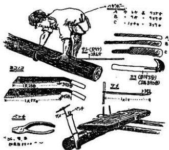
図2 山仕事道具
