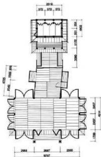
↑高木神社(上) 神殿・押殿平面図 1/300
