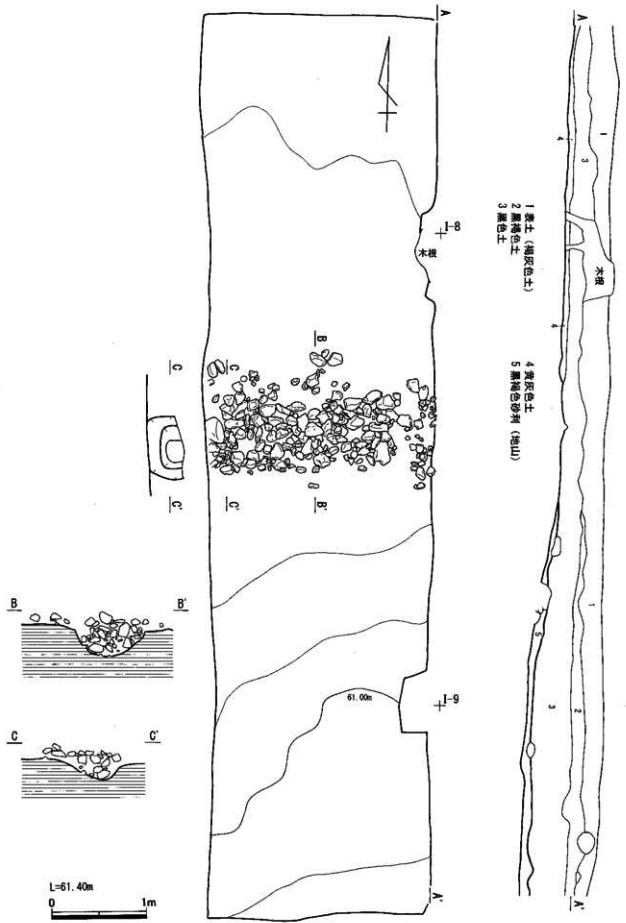
第7図 第12トレンチ実測図
