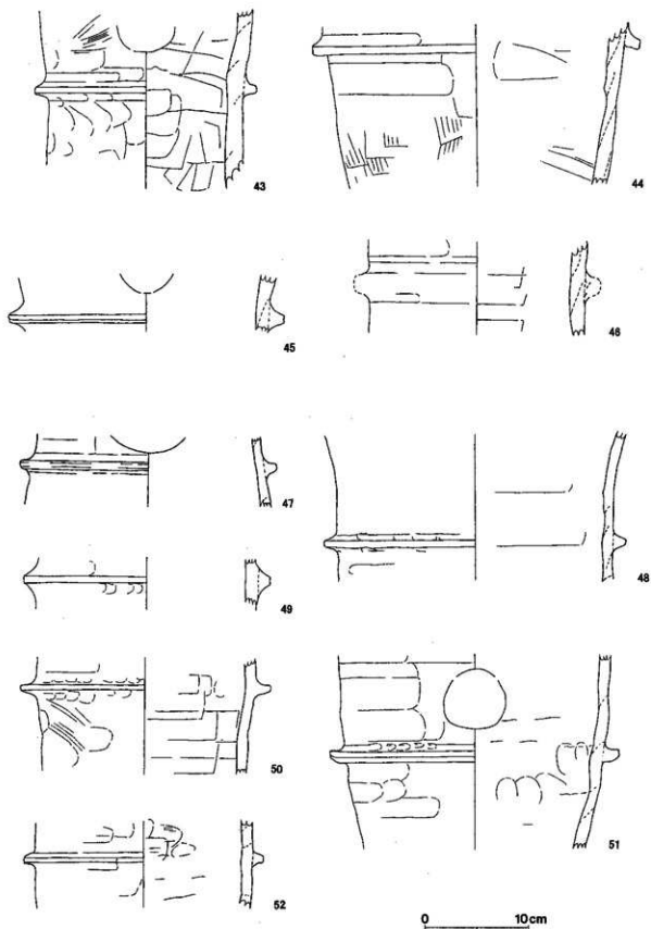
第13图 吉岡大塚古墳出土土輪軸実測図(3)
