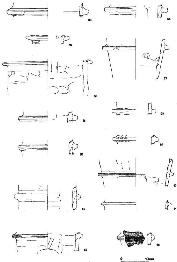
第14图 古岡大塚古墳出土輪突測図(4)
