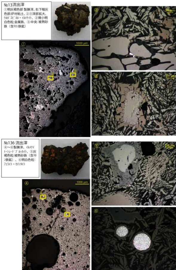
図54 炉底滓・流出滓の顕微鏡写真
