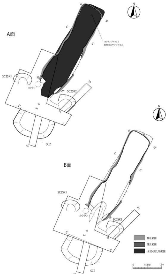
図47 2号木炭炭跡(1)
