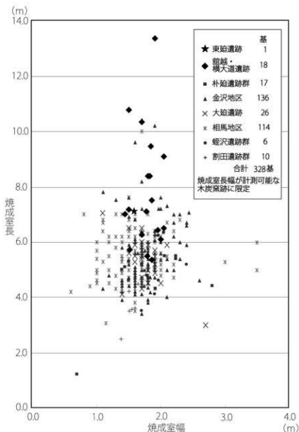
図59 焼成室長幅散布図
