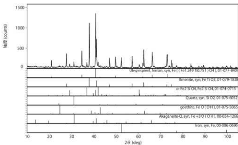
X線回折結果 (供試料:No.5)
