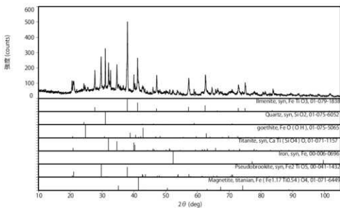
X線回折結果 (供試料:No.46)
