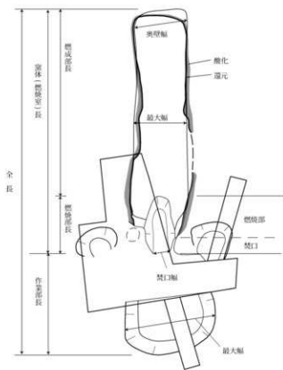
木炭窯跡
