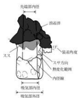
羽口
