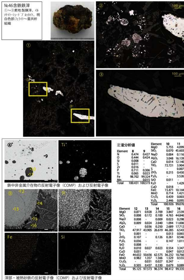
図56 含鉄鉄滓の顕微鏡写真・EPMA調査結果(2)
