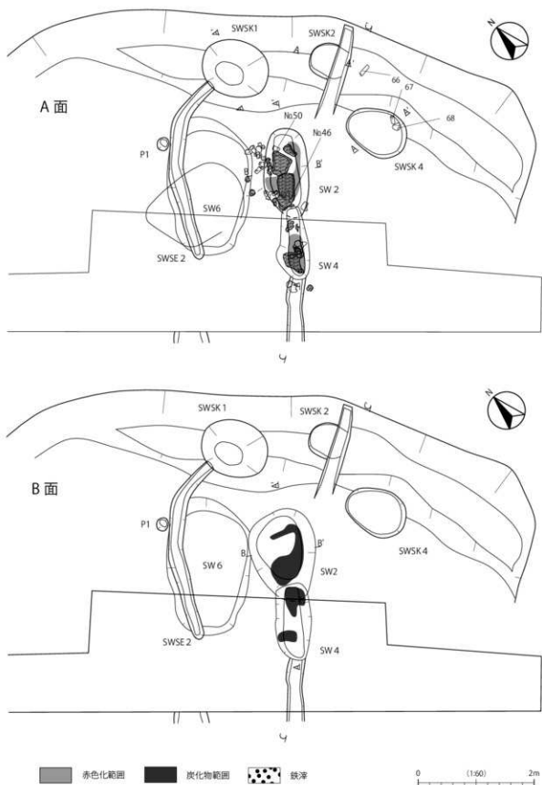
図17 2号製鉄炉跡(1)
