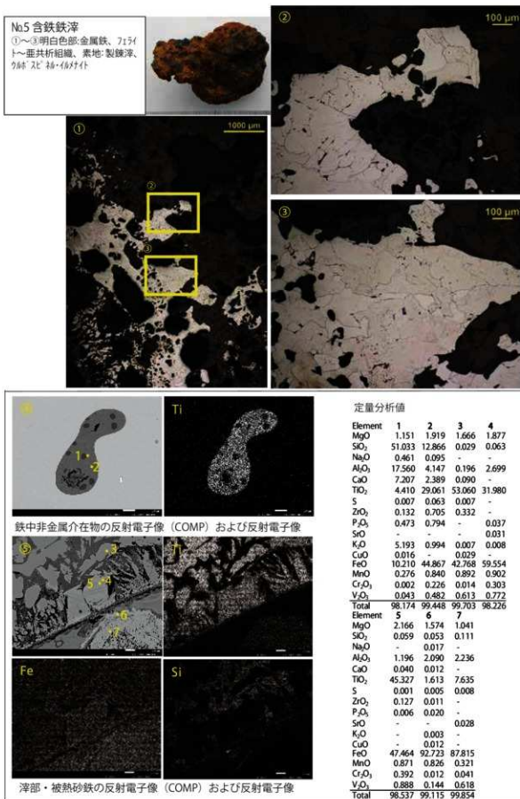
図55 含鉄鉄滓の顕微鏡写真・EPMA調査結果(1)
