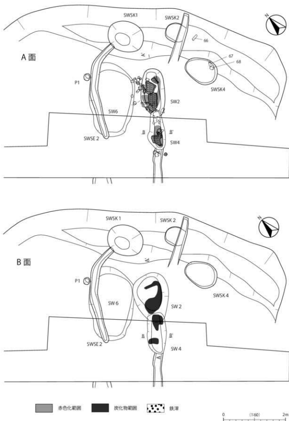
図23 4号製鉄炉跡(1)
