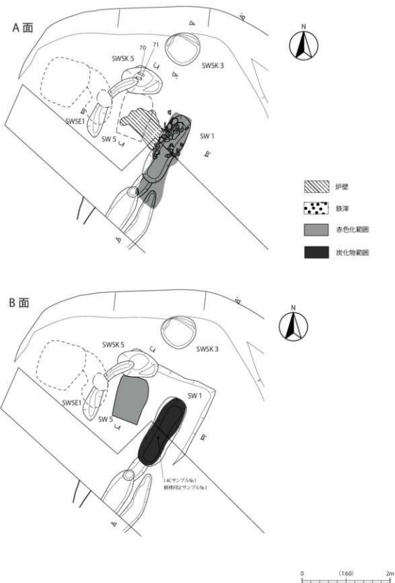
図10 1号製鉄炉跡(1)
