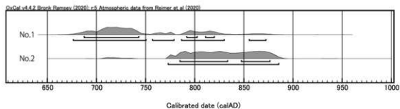
図 58 暦年較正結果
