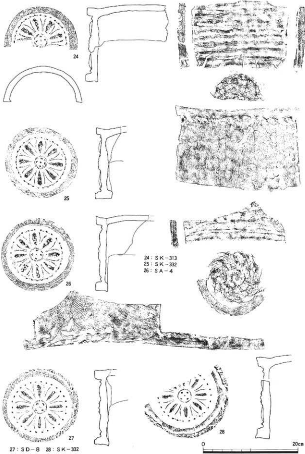
第106图 出土瓦实测图一4 (1/4)
