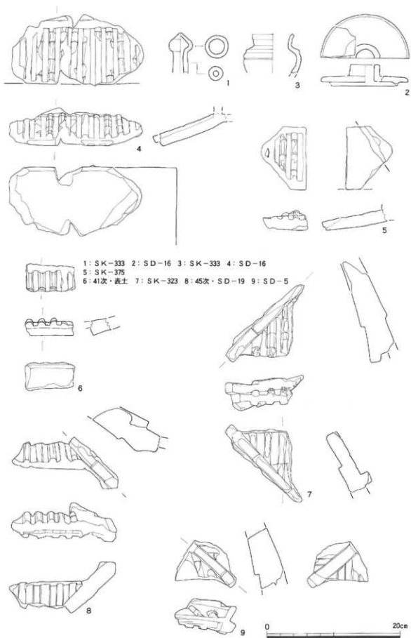
第129图 出土瓦塔实例图一 (1/4)
