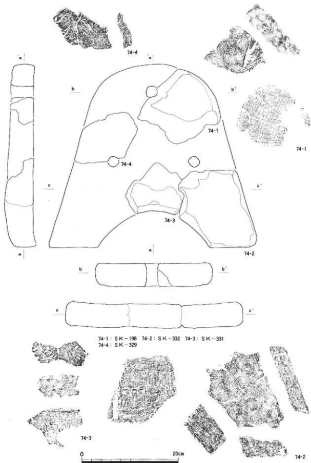
第128图 出土瓦実測図-26 (1/4)
