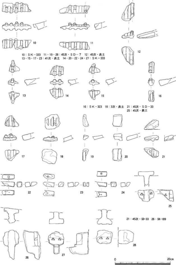
第130图 出土瓦塔实测图-2 (1/4)
