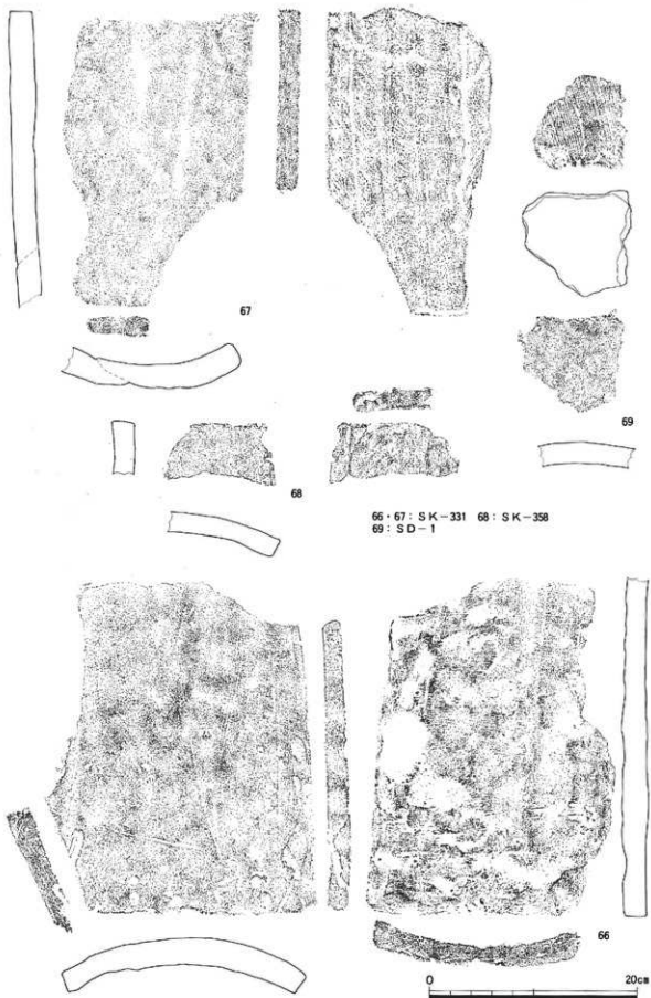
第126图 出土瓦実測图-24 (1/4)
