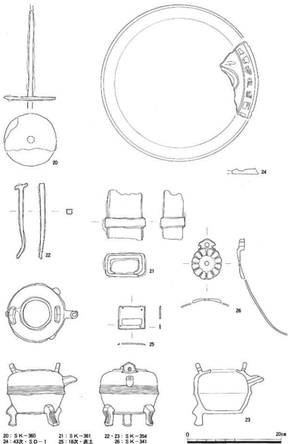
第134图 出土金属器实测图—2 (1/2)
