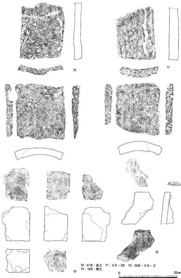
第127図 出土瓦実測図-25 (1/4)
