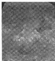
支笏軽石流堆積物の集中
