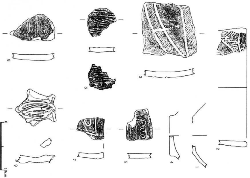
第6圖 出土遺物実測図
