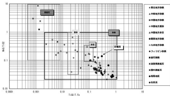
図5 砂鉄と鉄鉱石原料の酸化チタン (TiO 2 ) と酸化マンガン (MnO) との関係
