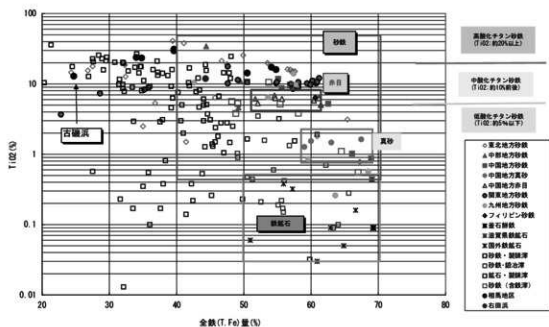
図3 砂鉄と鉄鉱石原料の全鉄量と酸化チタン量との関係
