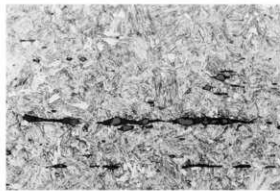
写真 43 資料 No. 5 L断面鉄組織写真×400 (1)
