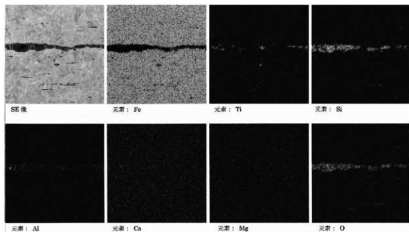
写真 50 サンプル5 L マッピング分析結果 × 800
