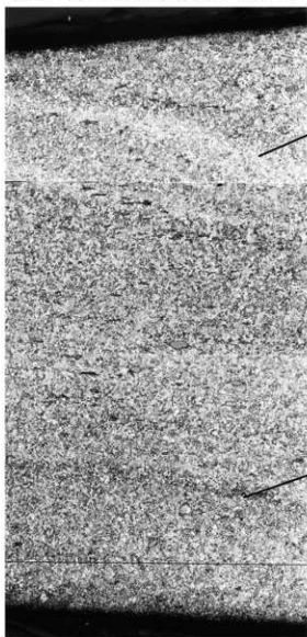
写真 37 資料 No. 5 の C 断面組織写真×100
