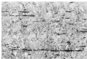
写真 44 資料 No. 5 L断面鉄組織写真×100 (2)
