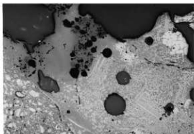
写真 23 資料 No. 3 顕微鏡写真 \times 100 (2)
