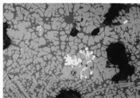
写真14 資料No.1 顕微鏡写真×400 (1)
