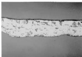
写真 18 資料 No. 2 顕微鏡写真 \times 400 (1)
