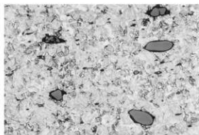
写真 39 資料 No. 5 C断面鉄組織写真×400 (1)
