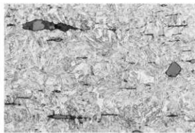
写真 45 資料 No. 5 L断面鉄組織写真×400 (2)
