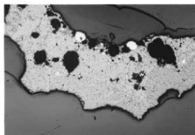
写真15 資料No.1 顕微鏡写真×100 (2)
