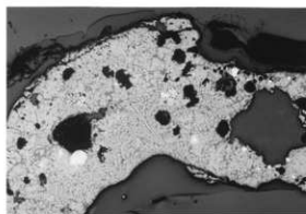
写真13 資料No.1 顕微鏡写真×100 (1)
