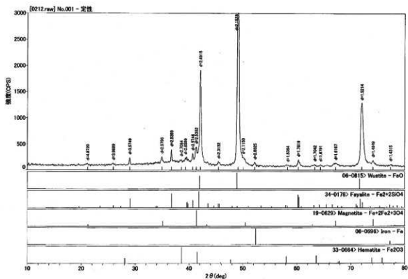
図7 X線回折チャート1 (資料 No. 1)
