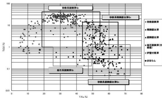
図1 出土鉄滓類の全鉄量と二酸化チタン量の分布図
