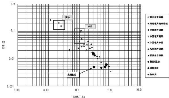
図6 砂鉄中の酸化チタンとバナジウムの分布図
