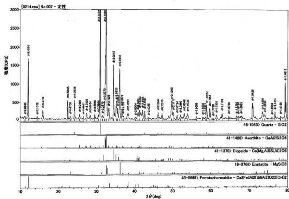
図9 X線回折チャート3 (資料 No. 7)
