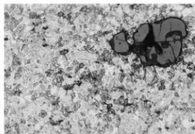
写真 41 資料 No. 5 C断面鉄組織写真×400 (2)
