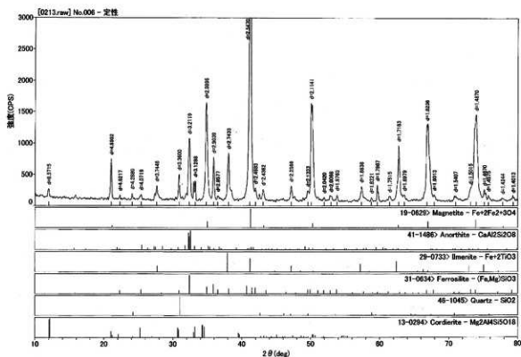
図8 X線回折チャート2 (資料 No. 6)
