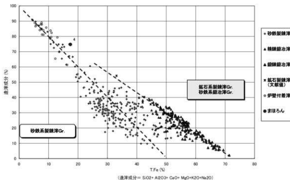
図2 製錬滓と鍛冶滓の分類
