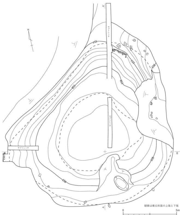
図6 巨勢山281号墳墳丘測量図
