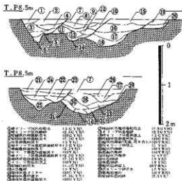
fig. 7 SD-14断面図
