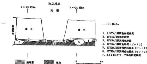
図3 Na.2地点遺構断面図(1:40)
