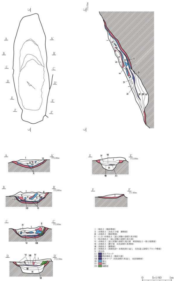
第5図 X次調査須惠器窯
