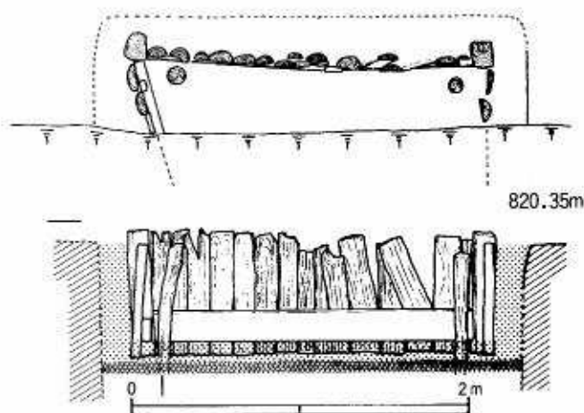
第3図 木組樹
