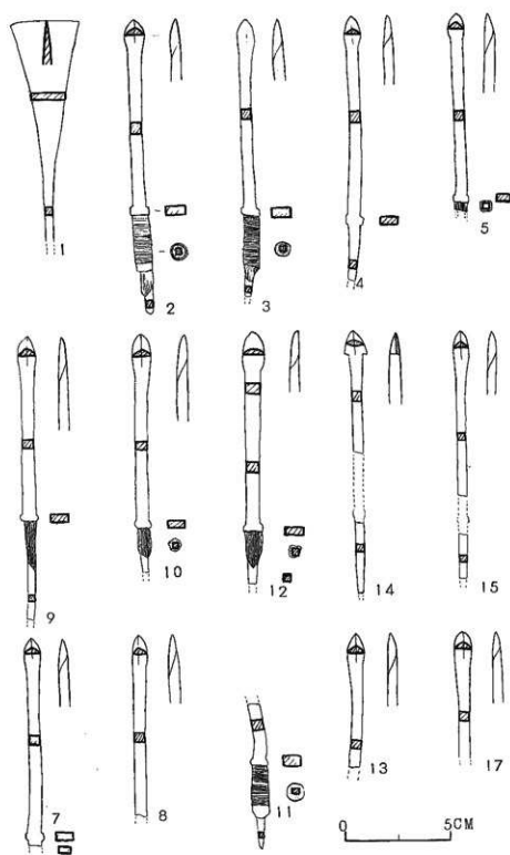
图12 铁钉实测图
