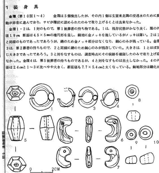
図10 装身具類実測図
