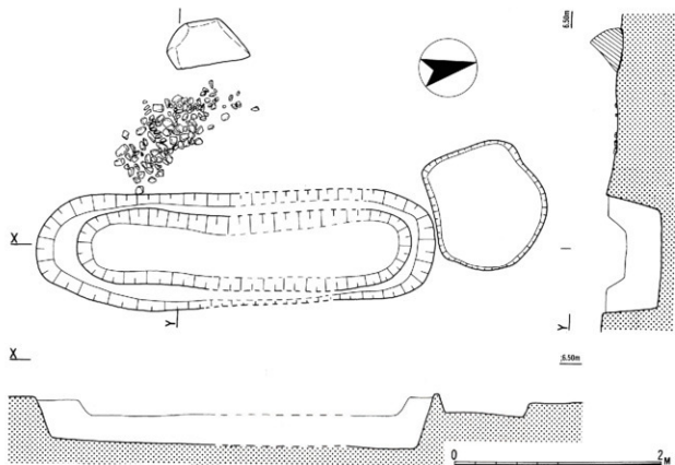
主体部実測図 (1:40)
