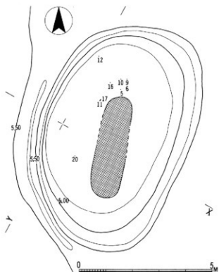
調査後墳丘実測図 (1:100)
