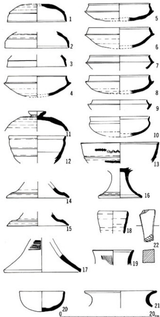
出土遺物実測図 (1:4)
