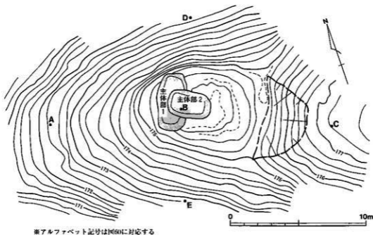
図59 巨勢山409号墳 墳丘 測量図 (S=1/200)
