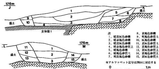
図65 巨勢山409号墳 主体部2 断面図 (S.=1/30)
