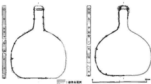
図54 巨勢山408号墳 出土鐘 復原図 (S=1/4)
