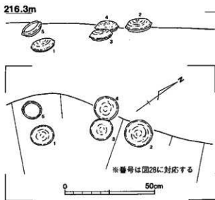
図26 巨勢山407号墳 墳丘 遺物出土状態 (S-1/15)
