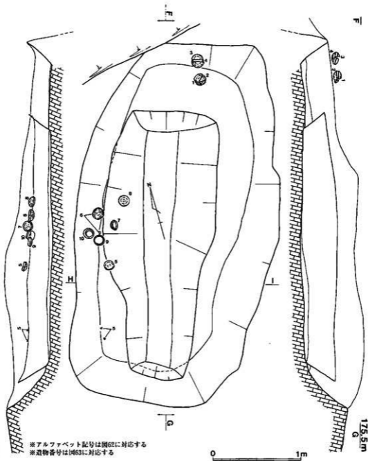
図61 巨勢山409号墳 主体部1 平面・立面図 (S=1/30)
