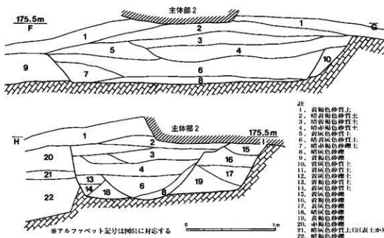
図62 巨勢山409号墳 主体部1 断面図 (S=1/30)
