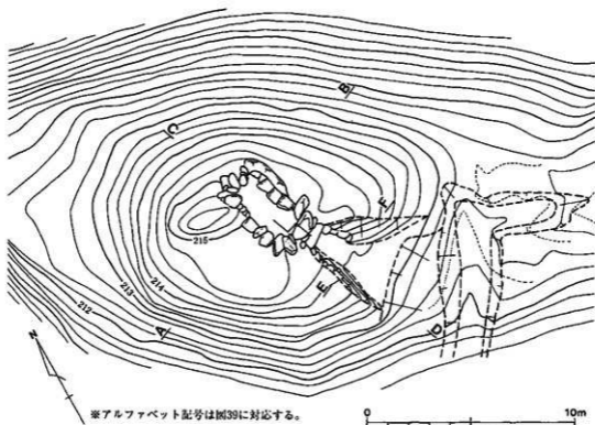
図38 巨勢山408号墳 墳丘 測量図 (S=1/200)
