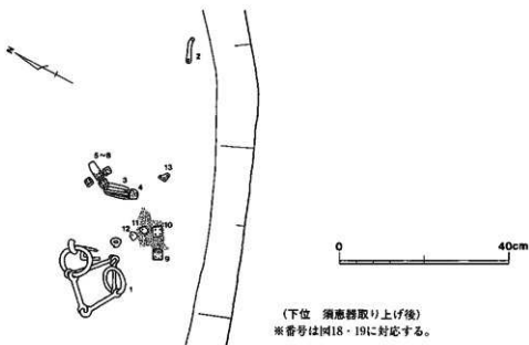
図15 巨勢山371号墳 主体部2 遺物出土状態2 (S=1/10)
