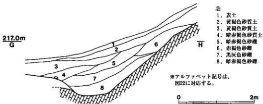
図23 巨勢山407号墳 東側周溝 断面図 (S 1 =1/50)
