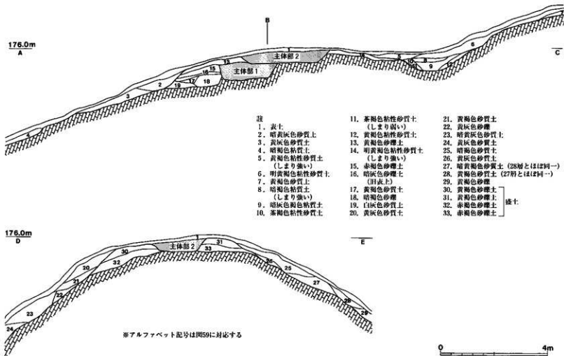
図60 巨勢山409号墳 墳丘 断面図 (S=1/100)
