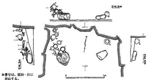
図27 巨勢山407号墳 追葬面 遺物出土状態 (S=1/30)
