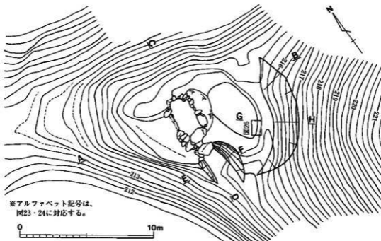
図22 巨勢山407号墳 墳丘 測量図 (S.=1/200)
