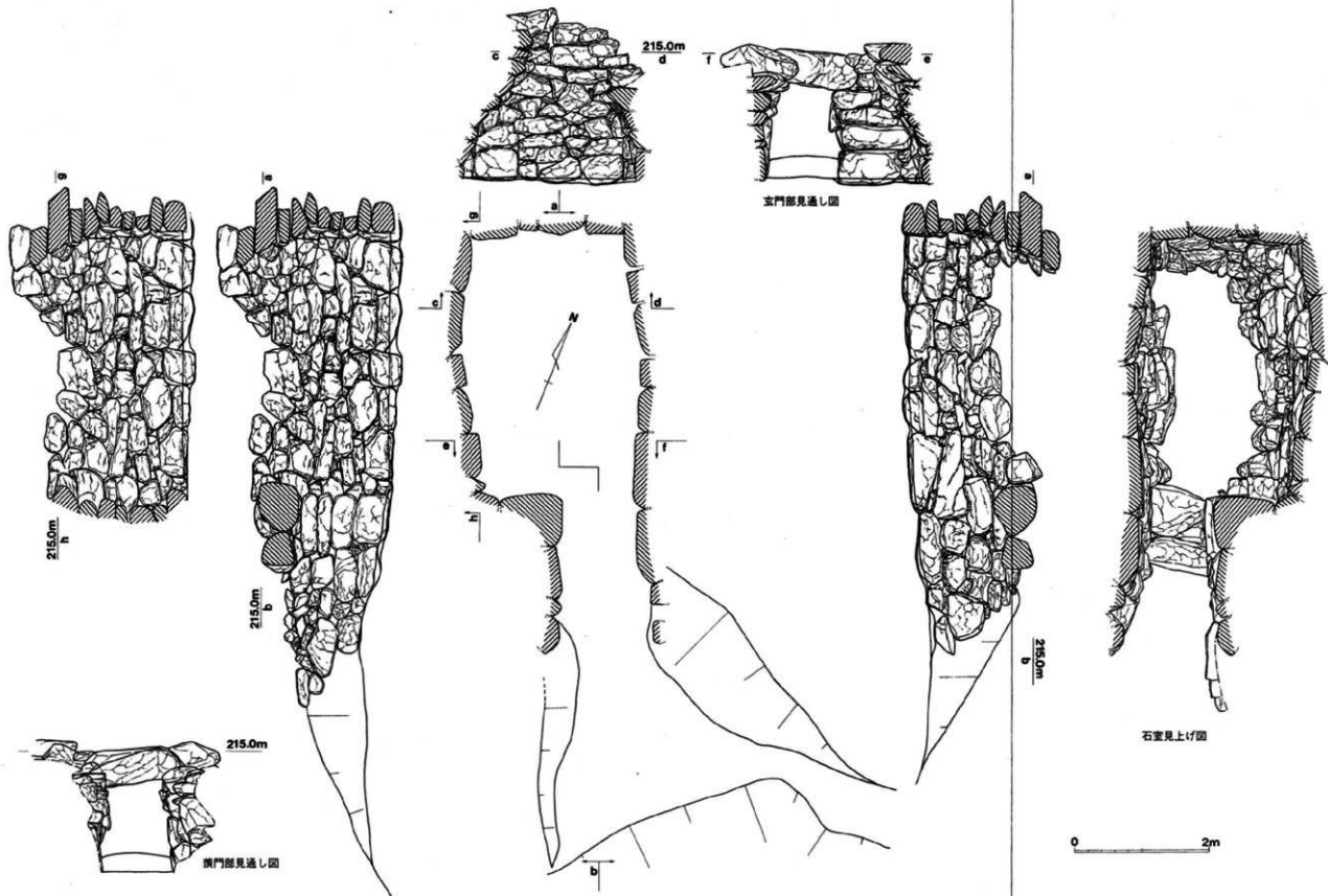
图40 巨勢山408号墳 横穴式石室 (S-1/80)
