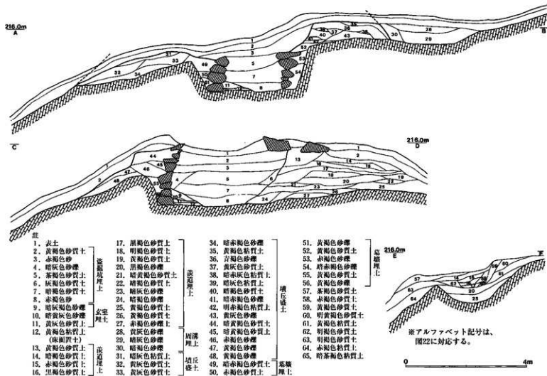
図24 巨勢山407号墳 墳丘・横穴式石室 断面図 (S=1/90)
