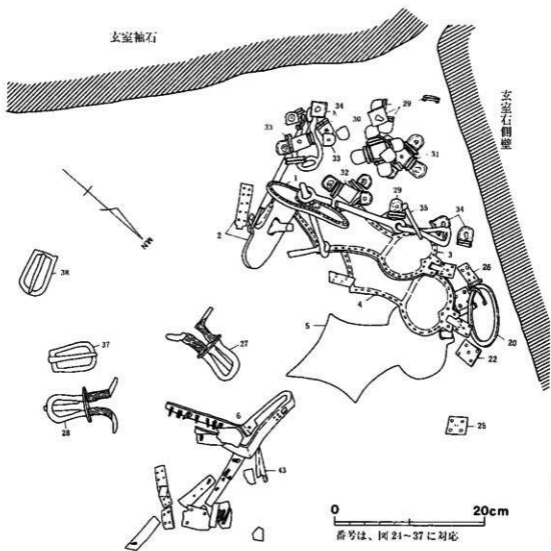
图20 巨勢山75号墳 玄室馬具出土状態 (S. = 1/5)
