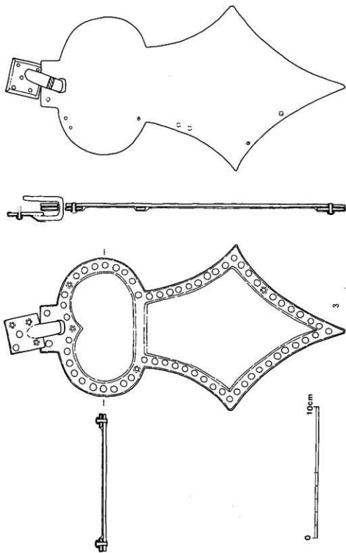
図26 巨勢山75号墳 玄室出土馬具（杏葉その1）（S. = 1/2）
