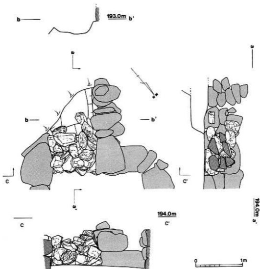
図17 巨勢山75号墳 石室 閉塞石 (S. = 1/40)
