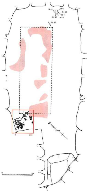
図19 巨勢山75号墳 石室床面の遺物 (S. = 1/30)
