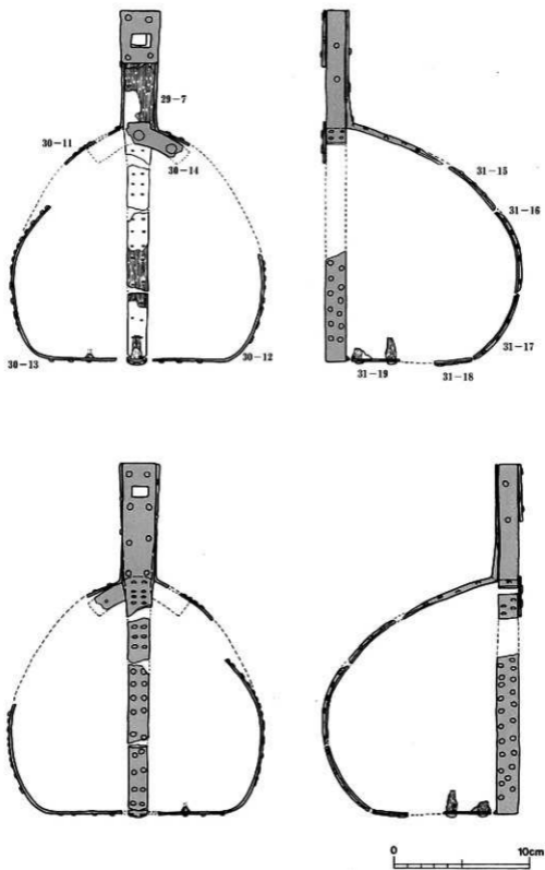
図33 巨勢山75号墳 玄室出土馬具（鑑復元図その2）（S. = 1 / 3）
