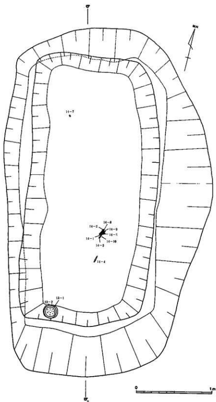
图 11 巨势山74号墳 主体部 2 平面图(S. =1/25)
