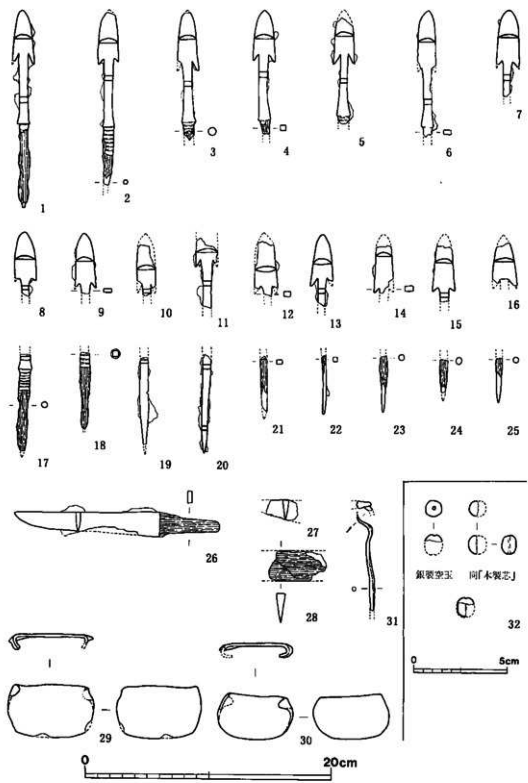
图38 巨勢山75号墳 出土鉄器・銀製品 (S. = 1 / 3 · 32は1 / 2)
