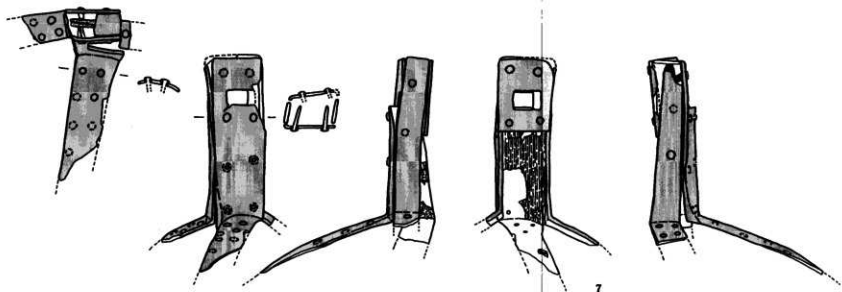
図29 巨勢山75号墳 玄室出土馬具（鏝その1）（S. = 1/2）
