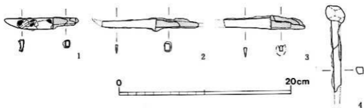
図10 巨勢山74号墳 主体部1 出土鉄製品 (S. = 1/3)
