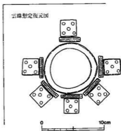
図34 〔勢山75号墳 玄室出土馬具（雲珠・雲珠復元図）（S. = 1/2・復元図はS. = 1/3）
