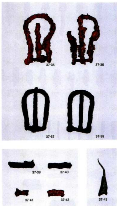
巨勢山75号墳 玄室出土馬具（鈎具・賁金具・飾金具） (s. 41/2)
