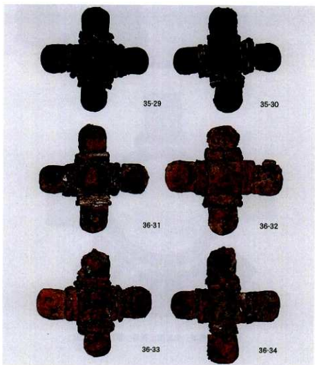
巨勢山75号墳 玄室出土馬具(鞍・辻金具) (s 1 ≒1/2)
