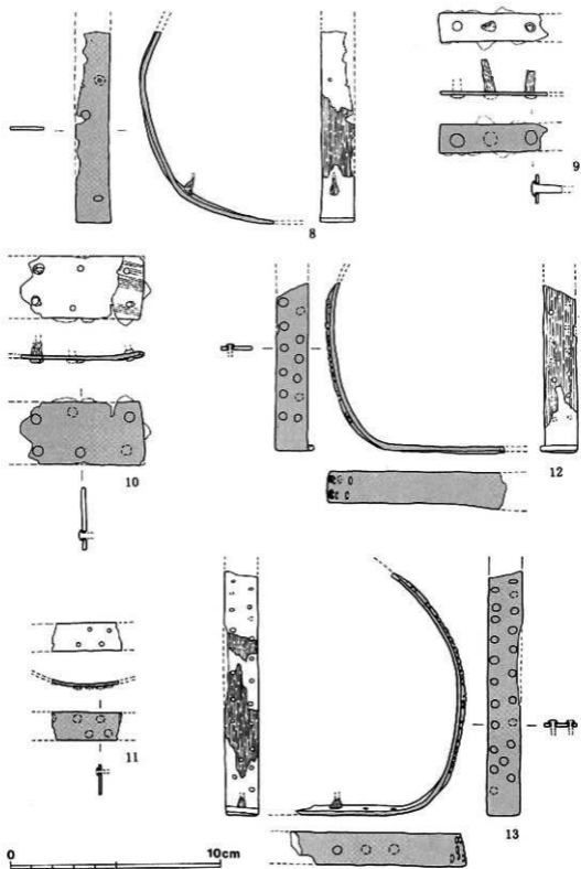
図30 巨勢山75号墳 玄室出土馬具（鍍その2）（S. = 1/2）
