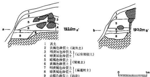
図18 巨勢山75号墳 石室 閉塞の状況 (S. = 1/40)
