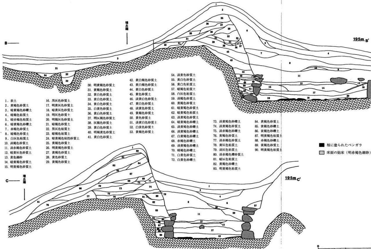
图 15 巨勢山 75号墳 墳丘断面土層図
