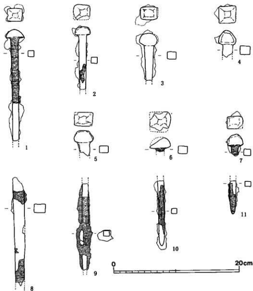
図39 巨勢山75号墳 出土鉄釘 (S. = 1/3)
