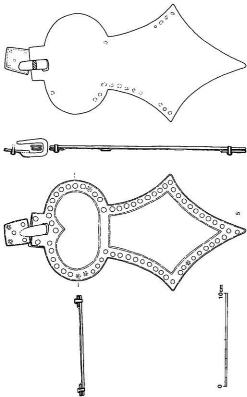
図28 巨勢山75号墳 玄室出土馬具（香葉その3）（S. = 1/2）
