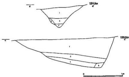
图 41 土坑 1 土层断面图 (S. = 1/30)
