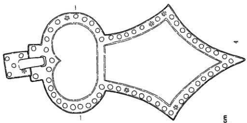
図27 巨勢山75分墳 支蓋出土馬具（各案その2）（S. = 1/2）
