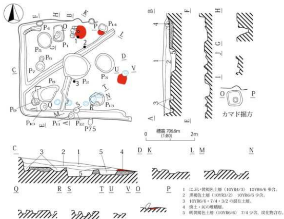
第4図 H1号住居址(1)
