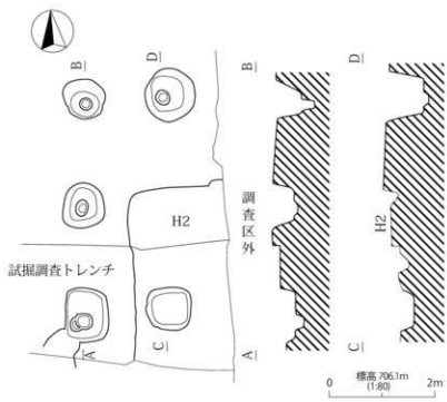
第13図 F3号掘立柱建物址
