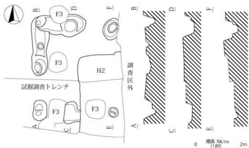
第14図 F4号掘立柱建物址
