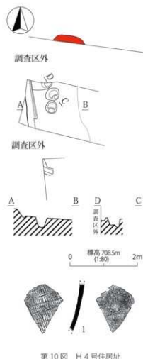
第10図 H4号住居址
