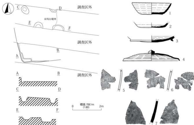
第9図 H3号住居址
