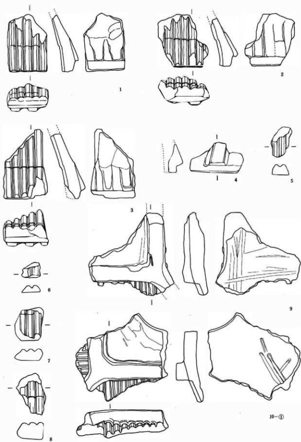
图159 船溪遗址出土瓦塔类陶器①(1:2)
