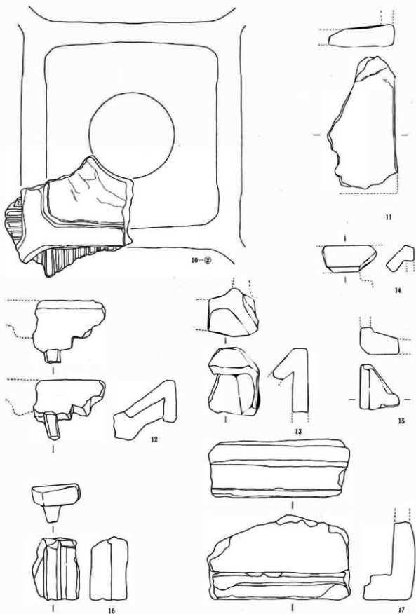
图160 榆溪遗址出土瓦塔实例图②(1:2)
