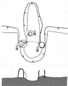
図96 FM I 区35号住居址カマド実測図(1:30)
