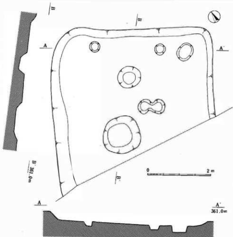
図77 FM 2区23号住居址実測図(1:60)
