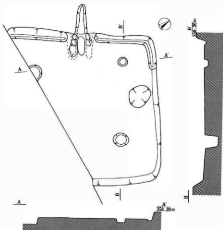
図104 FM3区1号住居址実測図(1:40)
