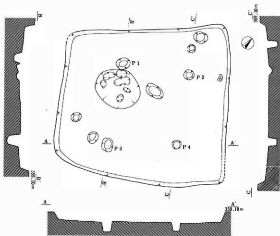
図85 FM1区9号住居実測図(1:60)
