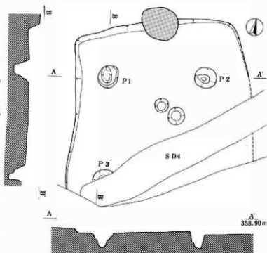
図109 FM1区7号住居址実測図(1:60)
