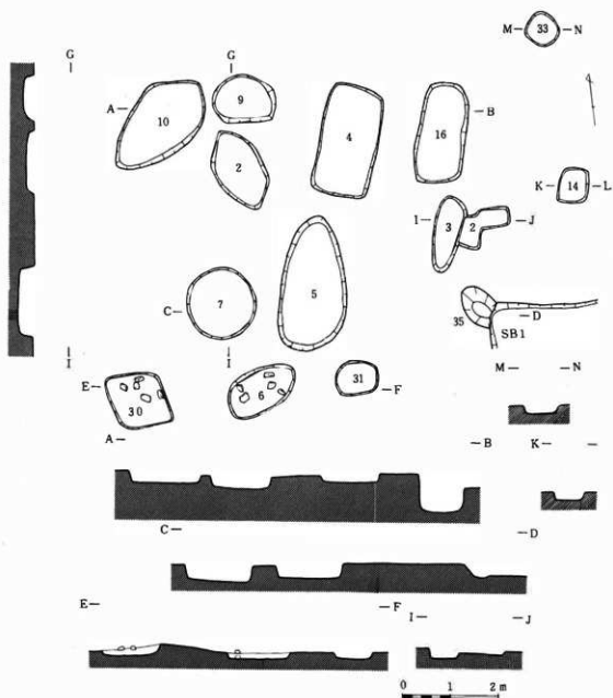
第35図 上部土坑群実測図 (1:80)
