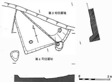
第8図 第3・4号住居址実測図
