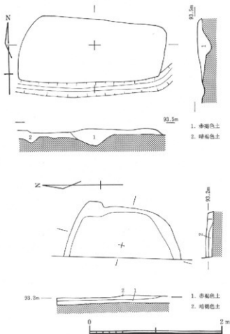
図-4 炉-1 (上)・炉-2 (下)
