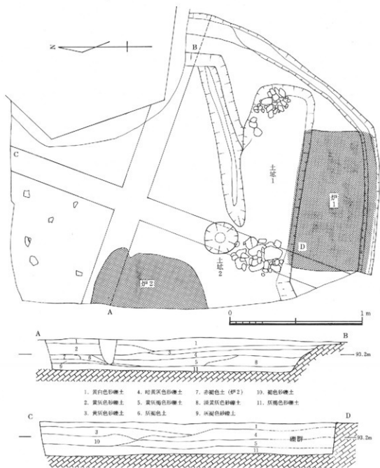
图-3 遺構平面図・断面図
