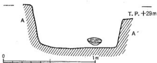
第51図 SE-1 平面図及び断面図
