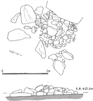
第48図 集石遺構-1 平面図及び立面図
