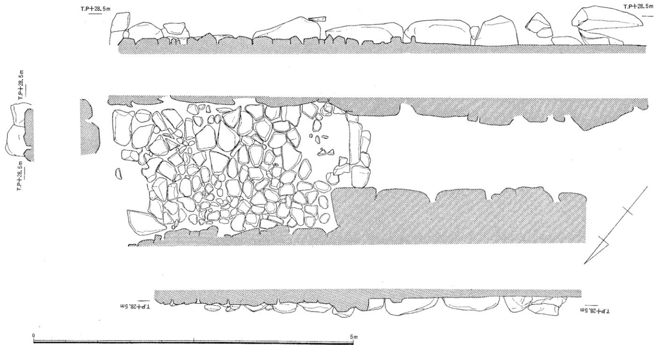
第17图 2号墳第1石室实测图
