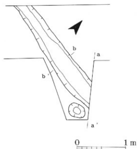
図3 溝1平面図
