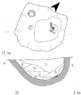
図8 土城1平面及び断面図
