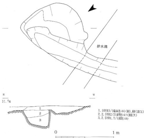
図 30 土城 4 平面及び断面図
