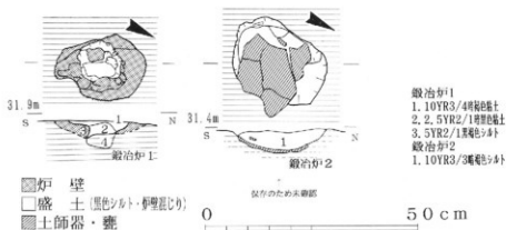
図31 鍛冶炉1, 2平面及び断面図
