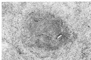
写真 2 4 鍛冶炉 1 検出状況
