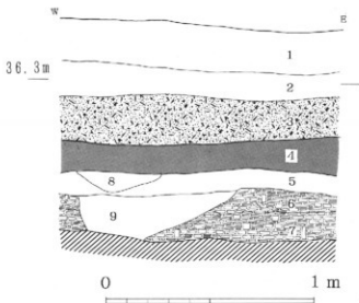
図7 地質断面図 (南側・溝2付近)
