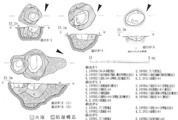
図15 鍛冶炉平面及び断面図
