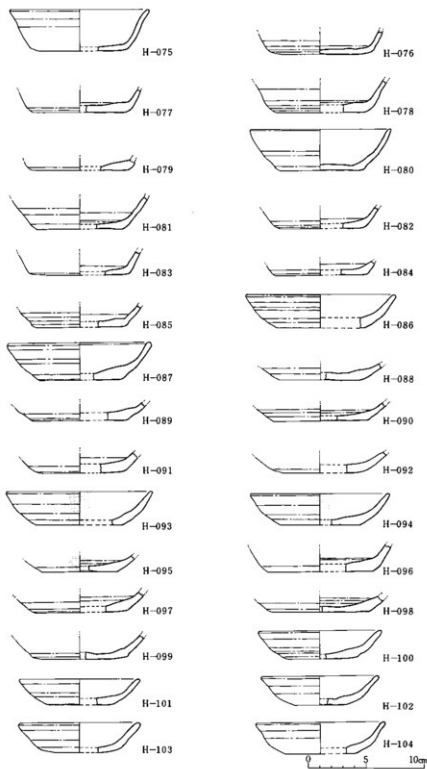
第32圖 土師器（杯）実測圖(3)
