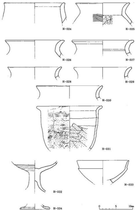
第41回 土師器 (徳・鉢・高杯) 実測図
