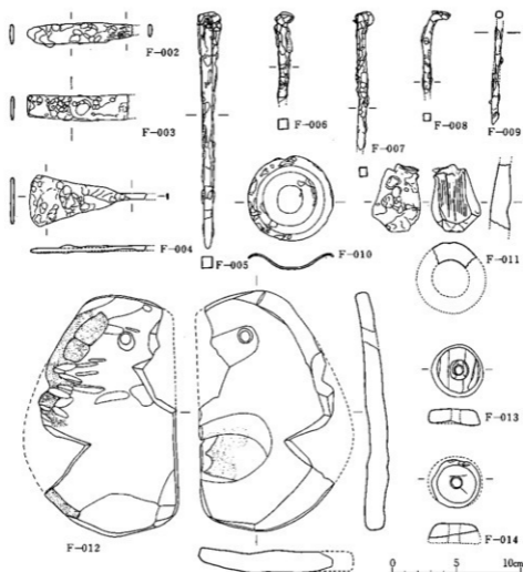
第46図 金属製品・石製品・繻羽口実測図
