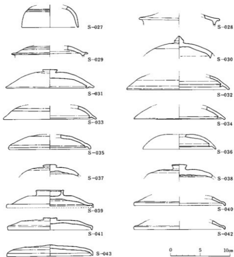
第26回 須恵器 (杯・蓋) 実測図
