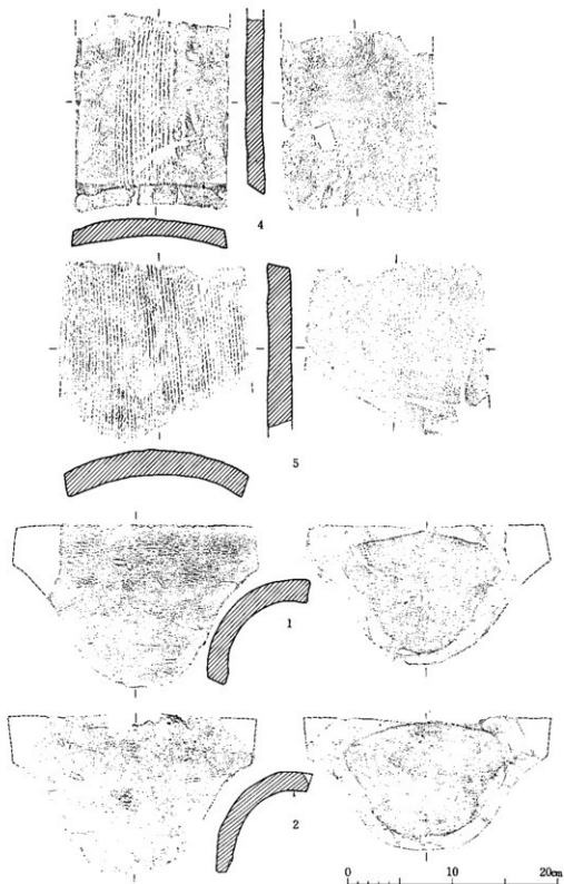
第25图 製斗瓦実測図(2)・面戸瓦実測図
