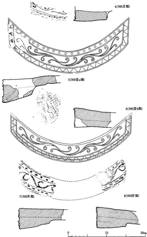
第188圖 軒平瓦実測圖(2)
