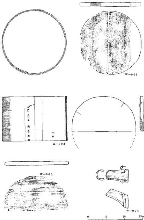
第47回 木製品実測図
