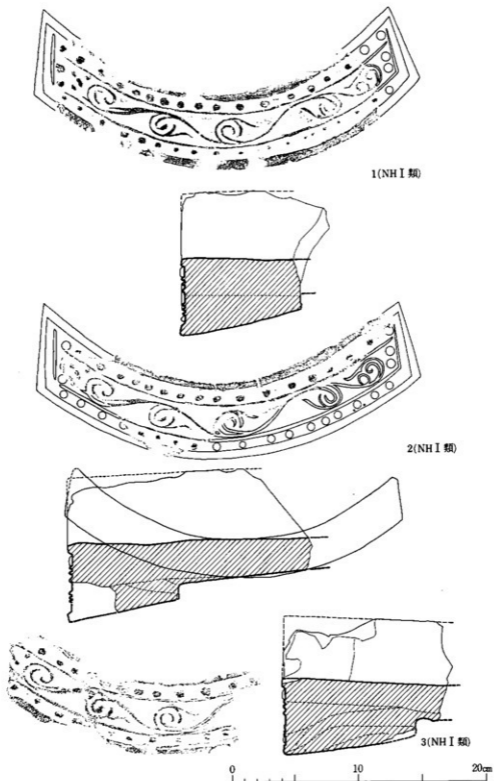
第17圖 軒平瓦実測圖(1)
