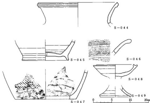
第29図 須恵器(甕・壺・高杯)実測図
