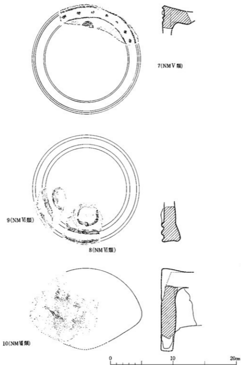
第16圖 軒丸瓦実測圖(3)
