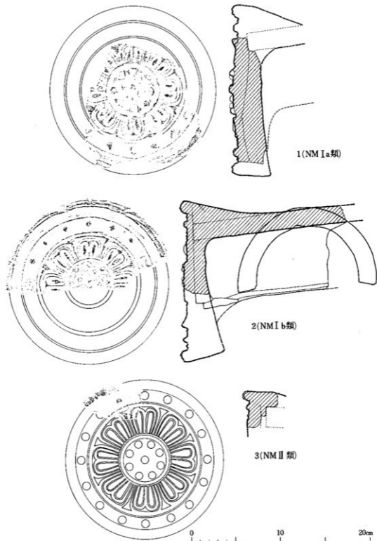
第14圖 軒丸瓦実測圖(1)
