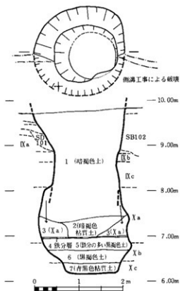
第7図 SE101実測図 S = 1 / 60
