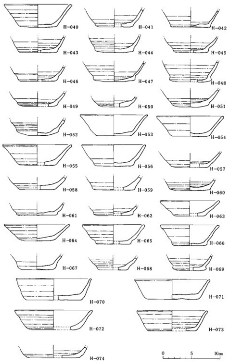
第31圖 土師器(杯)実測図(2)
