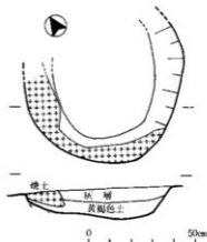
第5図 SX101実測図
