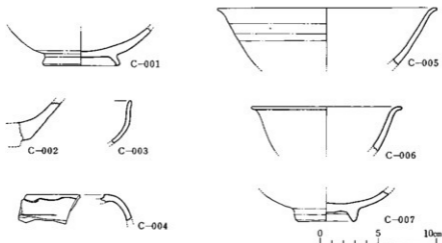
第44図 陶磁器実測図
