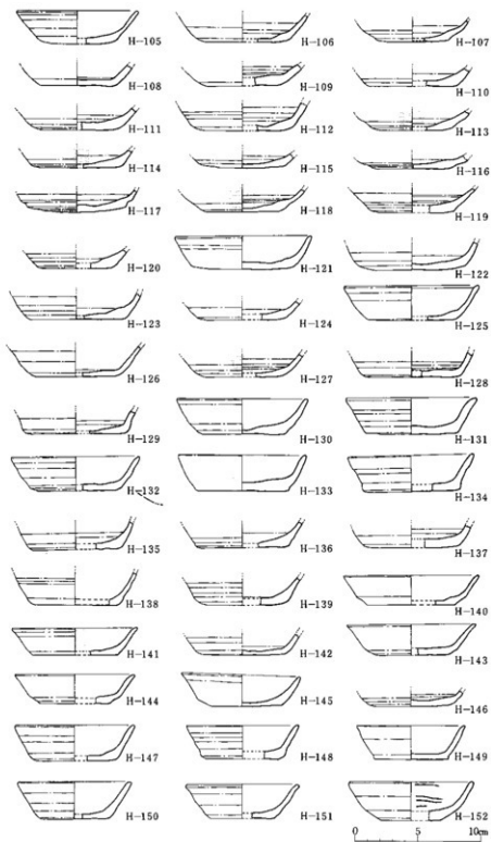
第33圖 土師器（杯）実測圖(4)
