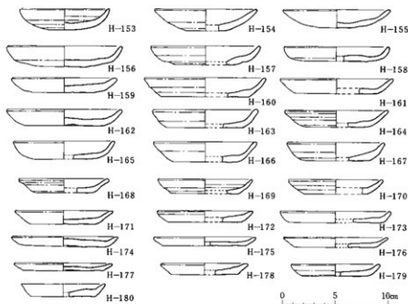
第34図 土師器(皿)実測図
