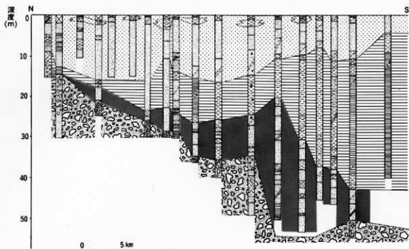
第 3 圖 滎尾平野地下地質模式断面圖 (南-北方向)
