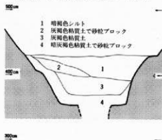
第22図 SE01土層セクション (1:40)
