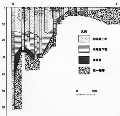
第 4 圖 滎尾平野地下地質模式断面圖 (東-西方向)
