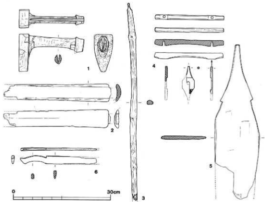
第3図 第2次調査出土の木製品 (S.=1/6)
