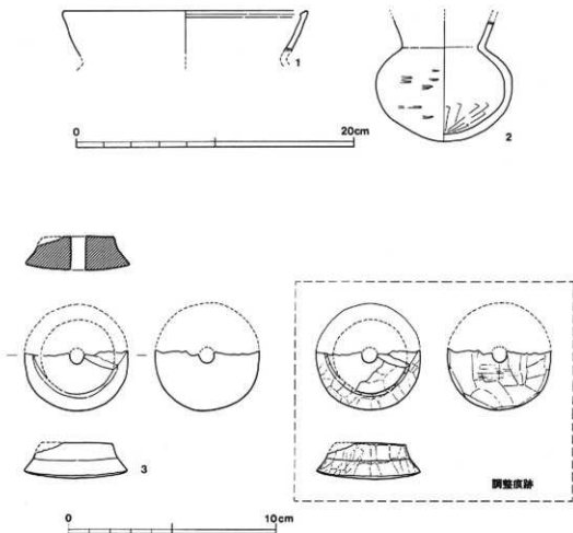
第5図 出土遺物1(1区第4層) 1・2 : S. = \frac{1}{3} , 3 : S. = \frac{1}{2}
