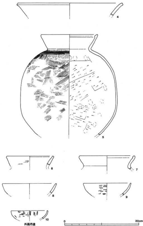
第6図 出土遺物2 (2区4a層(その1)) S. = 1/3
