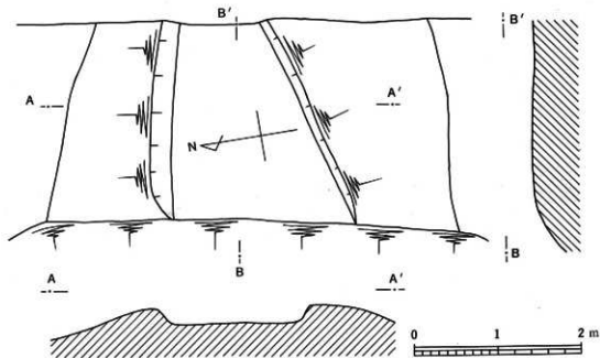
第9図 II-1号炉址実測図
