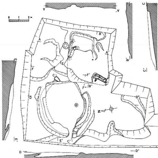
第22図 第四区北部地区遺構実測図
