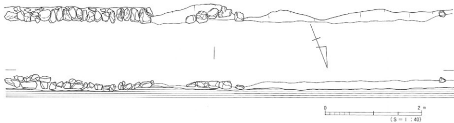
图15 列石平·立面图
