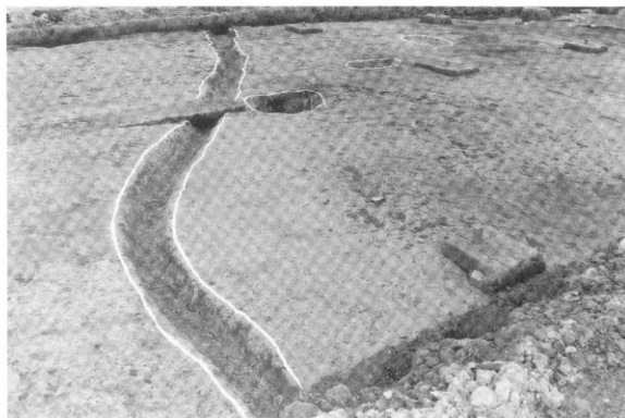
SD1（西より）
