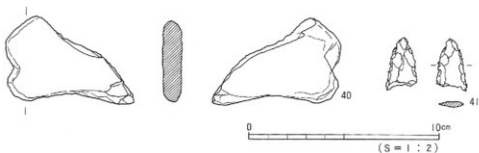
図20 2区出土石器
