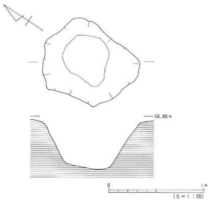
图26 土坑SK3
