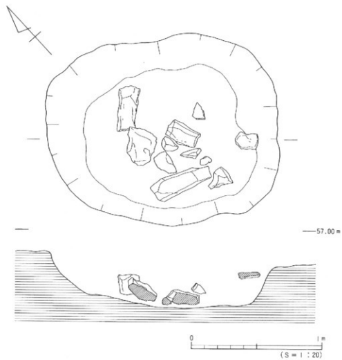
图24 土坑SK1
