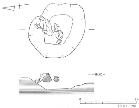
図29 土坑SK6
