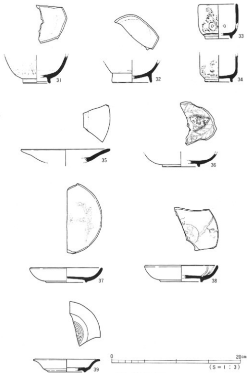
图19 2区出土磁器
