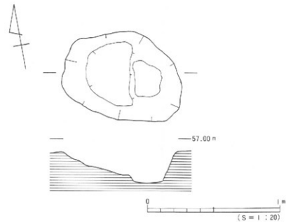
图25 土坑SK2
