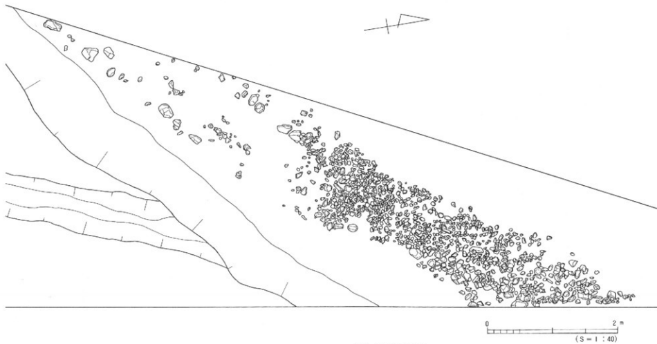
图16 2号暗渠平面图
