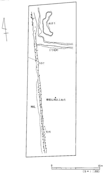
図30 4区遺構全測図
