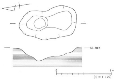
图27 土坑SK4
