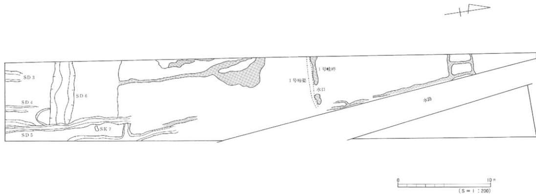
図4 1区調査全図
