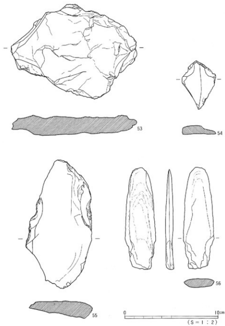
图32 4区出土遗物(2)
