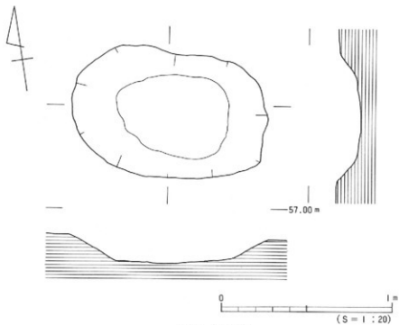
図28 土坑SK5
