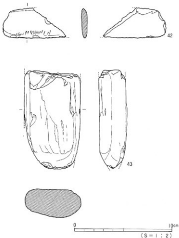
図22 3区出土石器
