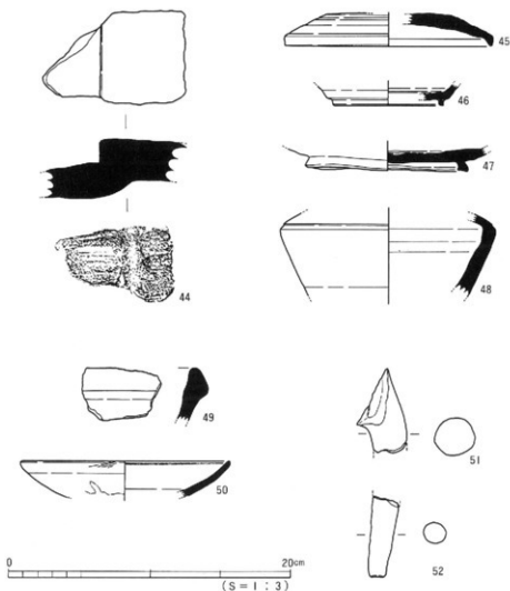
図31 4区出土遺物(1)
