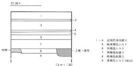
図2 層序模式図
