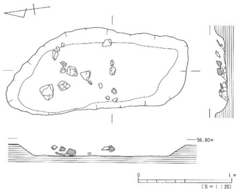
図21 土壌SK 8
