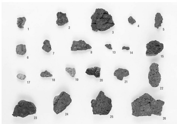
製鉄関連遺物（1）炉壁（1～8・17～26）・工具付着滓（13・14）・羽口（15） 写真中の数字は構成番号に対応する
