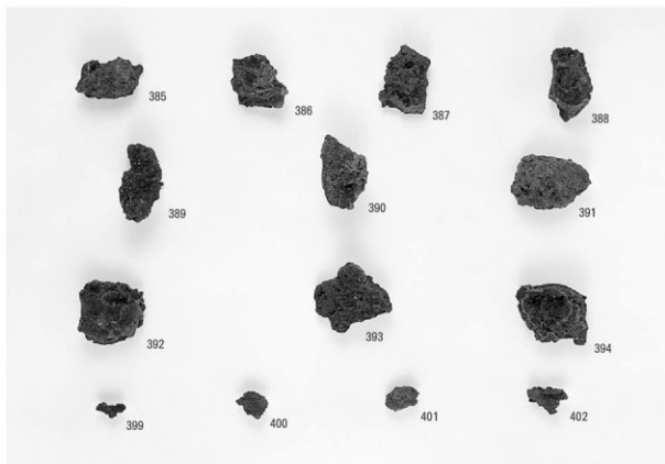
製鉄関連遺物 (22) 炉底塊 (385~394)・工具付着滓 (399~402)
