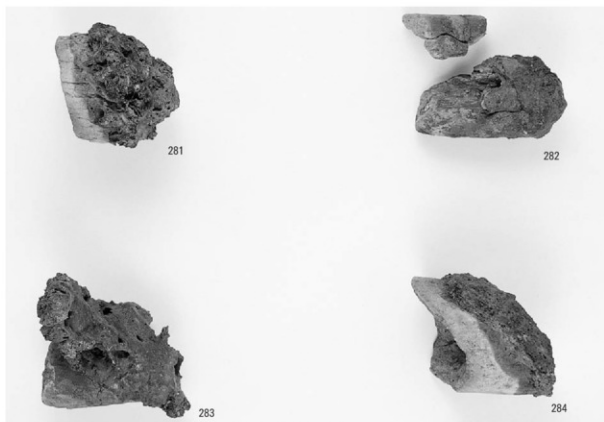
製鉄関連遺物 (14) 羽口
