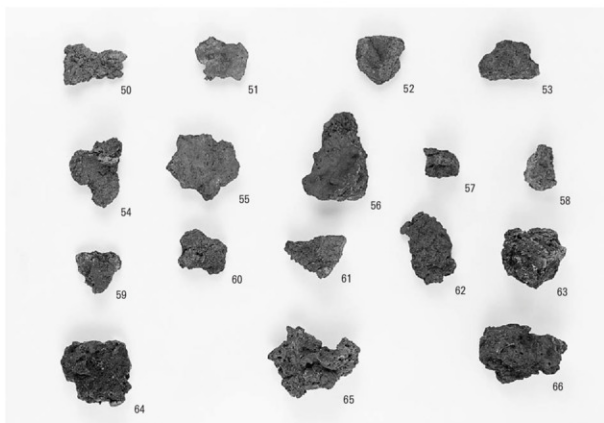
製鉄関連遺物（3）炉壁
