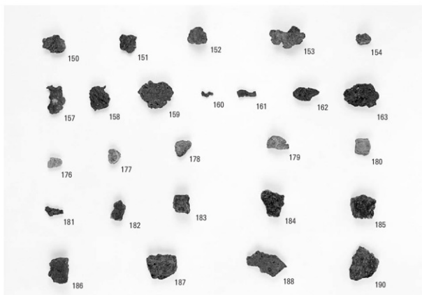
製鉄関連遺物 (7) 炉壁 (150・151・176~188・190)・炉内滓 (152・153)・炉底塊 (154) ・流動滓 (157~159)・単位流動滓 (160・161)・再結合滓 (162・163)
