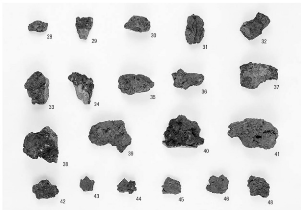
製鉄関連遺物（2）炉壁
