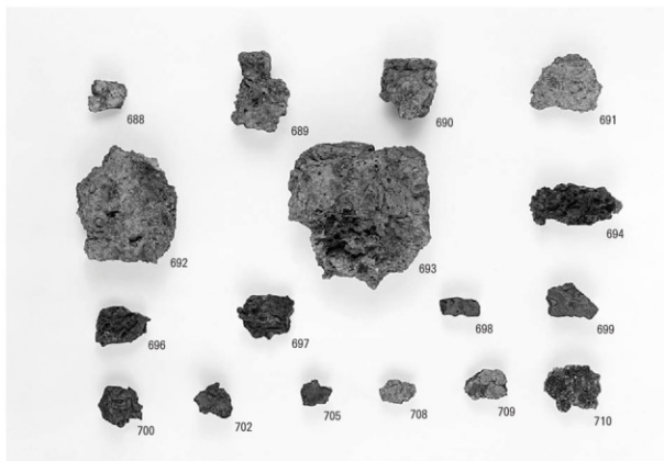
製鉄関連遺物 (24) 炉壁 (688~694・696・697・708~710) ・流出孔滓 (698) ・流出溝滓 (699) ・流動滓 (700) ・炉内滓 (702) ・再結合滓 (705)
