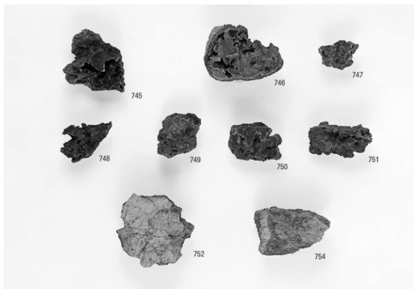
製鉄関連遺物 (29) 炉壁 (745~752)・羽口 (754)
