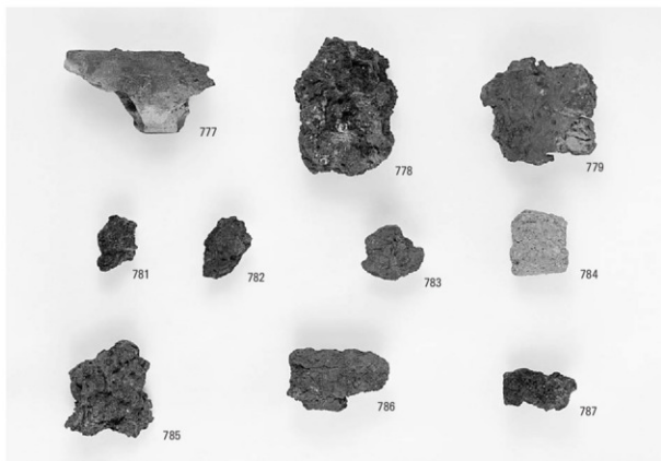
製鉄関連遺物 (32) 羽口 (777) ・炉壁 (778・779・781~786) ・マグネタイト系遺物 (787)
