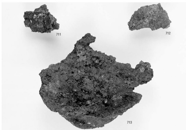
製鉄関連遺物 (25) 炉壁
