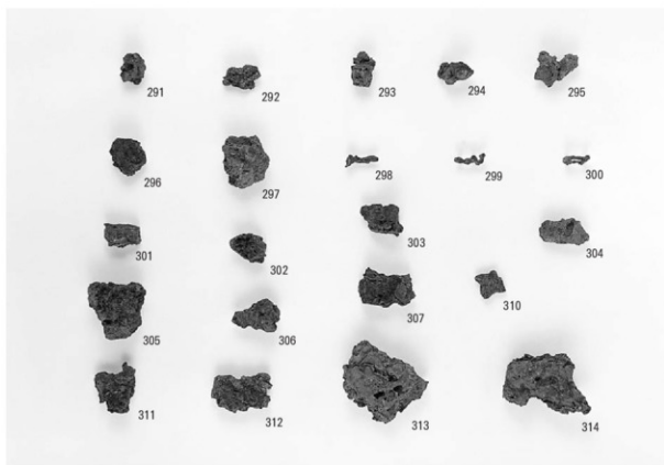
製鉄関連遺物 (17) マグネタイト系遺物(291~297)・単位流動滓(298~300)・流出孔滓(301~307)・流出溝滓(310~314)
