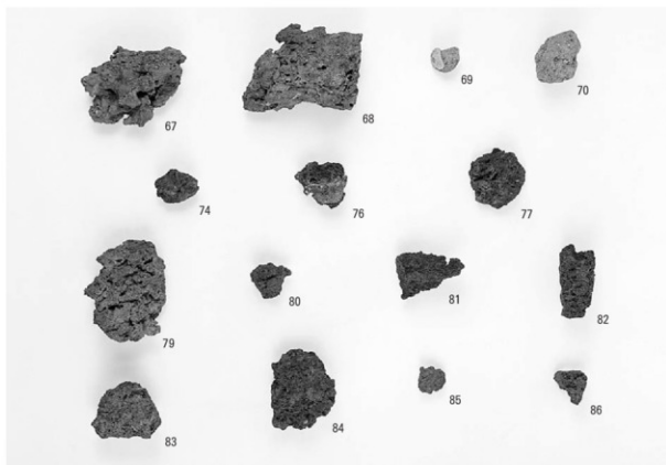
製鉄関連遺物（4）炉壁（67～70）・炉内滓（74・76・77・79～86）
