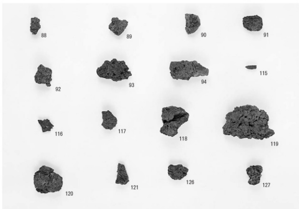
製鉄関連遺物 (5) 炉内滓(88~94)・黒鉛化木炭(115)・流動滓(116~121)・流出孔滓(126)・流出溝滓(127)
