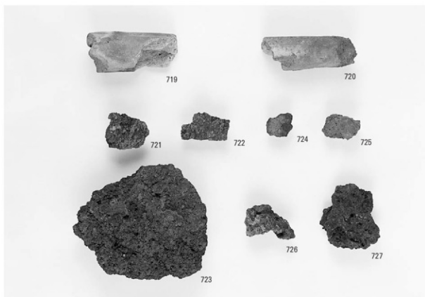
製鉄関連遺物 (27) 羽口 (719・720)・炉壁 (721・722・724~727)・再結合滓 (723)
