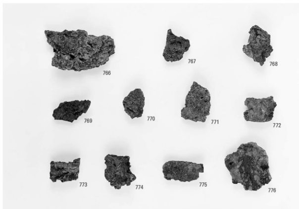
製鉄関連遺物 (31) 炉壁
