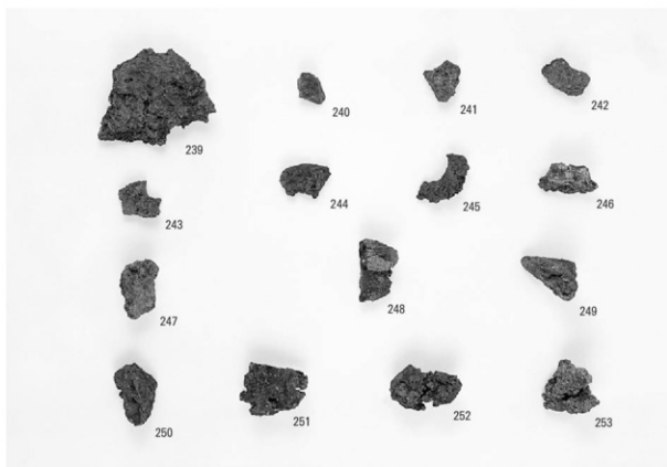
製鉄関連遺物 (11) 炉壁
