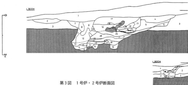
第3図 1号炉・2号炉断面図
