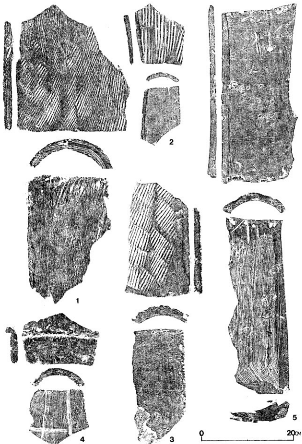
第8圖 丸瓦
