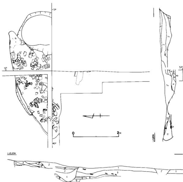
第2図 瓦窯跡平面図、断面図
