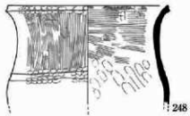
第37図 SX3平面・エレベーション図及び出土土器実測図
