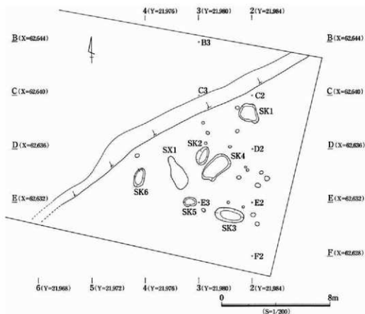
第5図 北区検出遺構配置図
