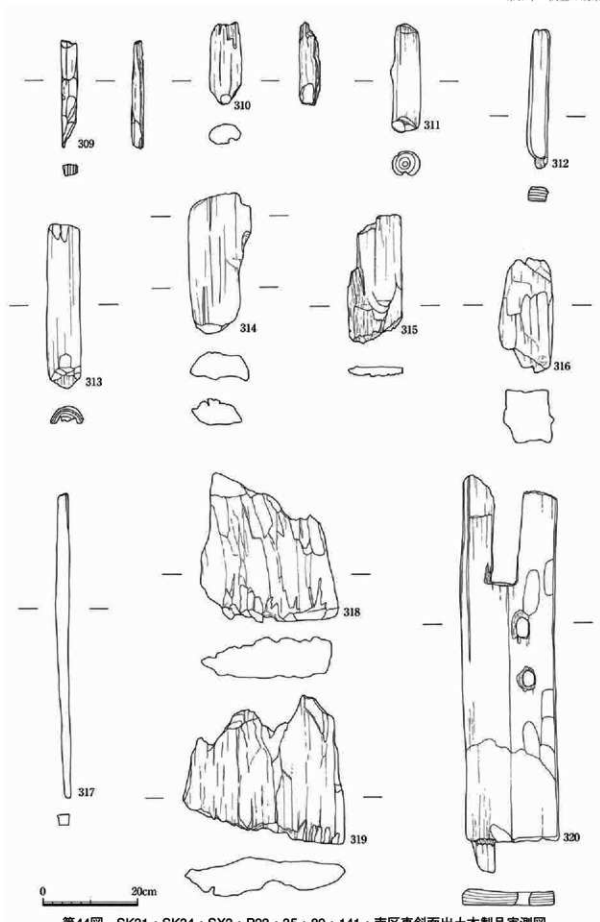
第44図 SK31・SK34・SX3・P23・35・89・141・南区東斜面出土木製品実測図
