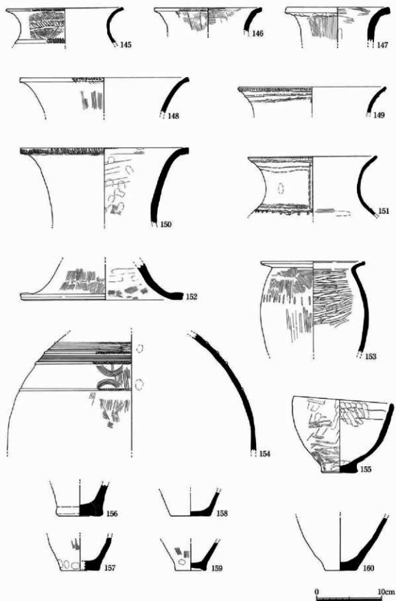
第26図 SK15出土土器実測図
