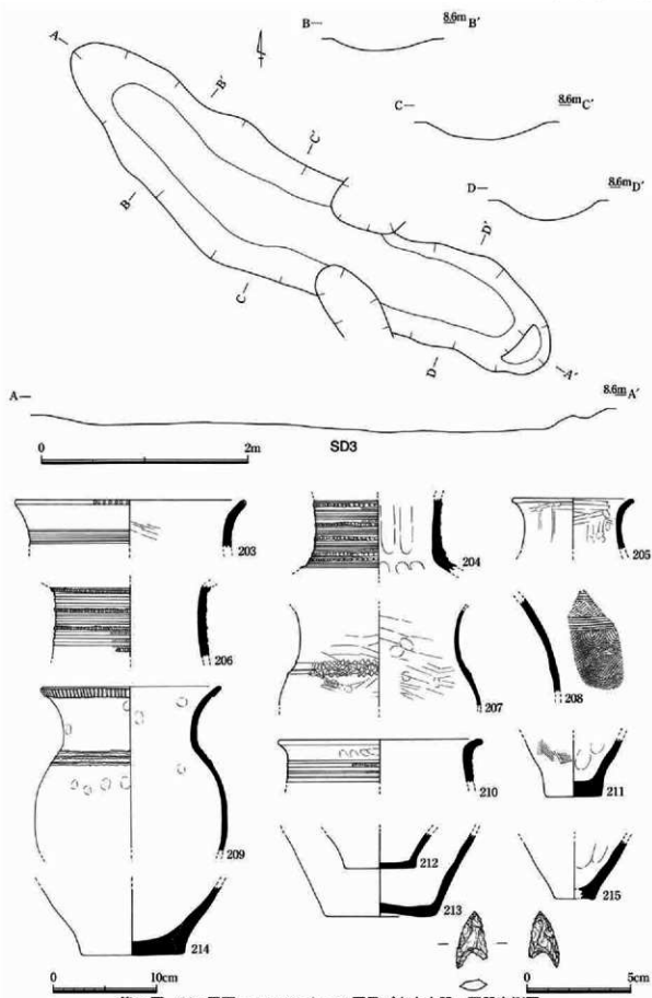
第36図 SD3平面・エレベーション図及び出土土器・石器実測図
