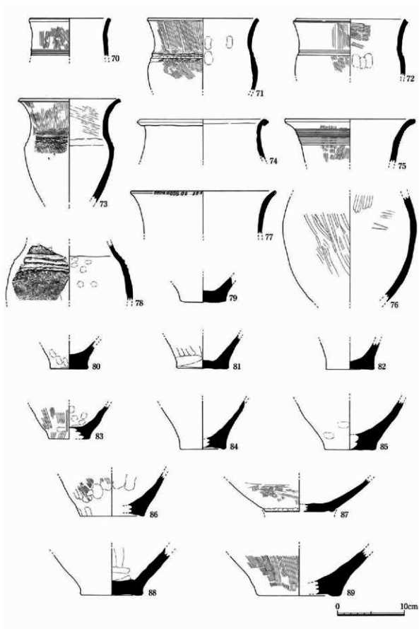
第14图 北区遺物包含層出土土器実測図 (2)
