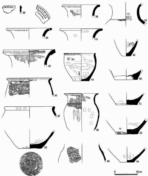
第12圖 旧河道出土土器実測圖
