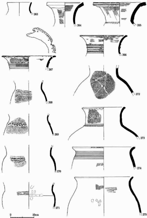
第39图 南区包含层出土土器实测图(2)
