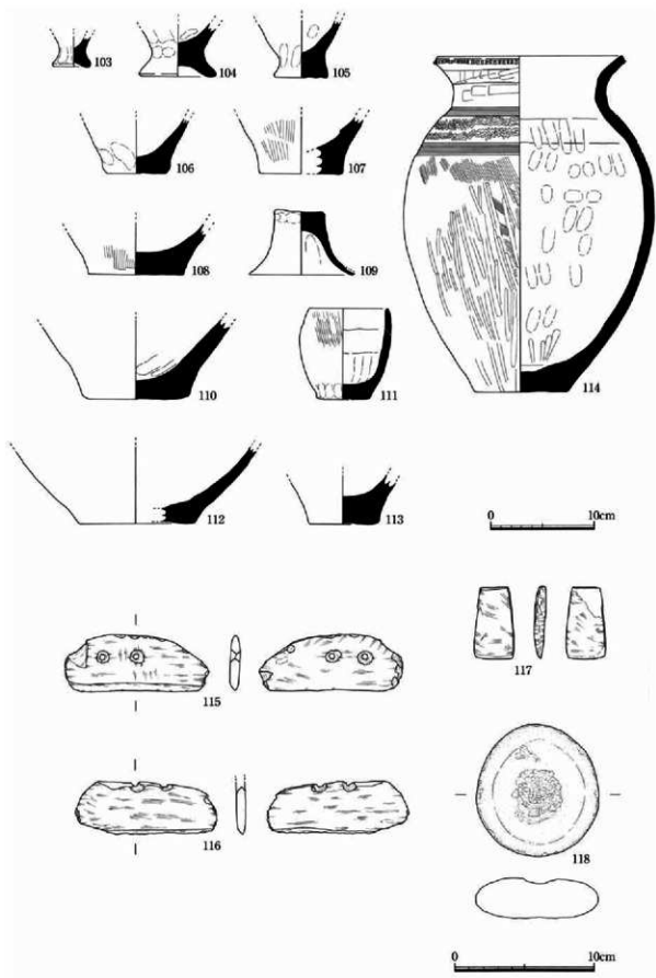
第16图 北区遗物包含層出土土器・石器実測図
