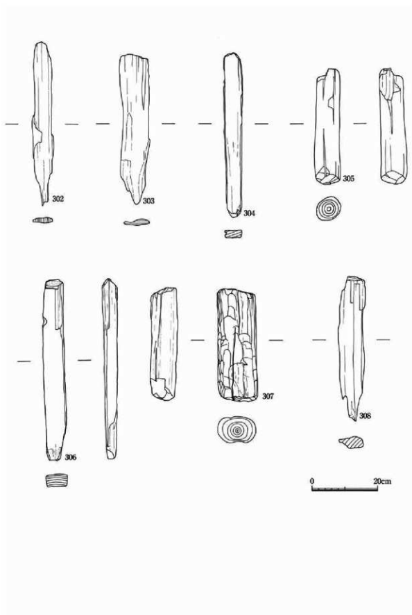
第43图 SK13·SX3·SD3·南区东斜面出土木制品实测图
