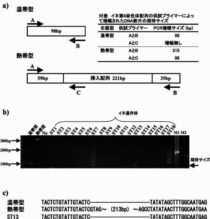
図6 イネの第6染色体領域の構造多型とPCR解析
