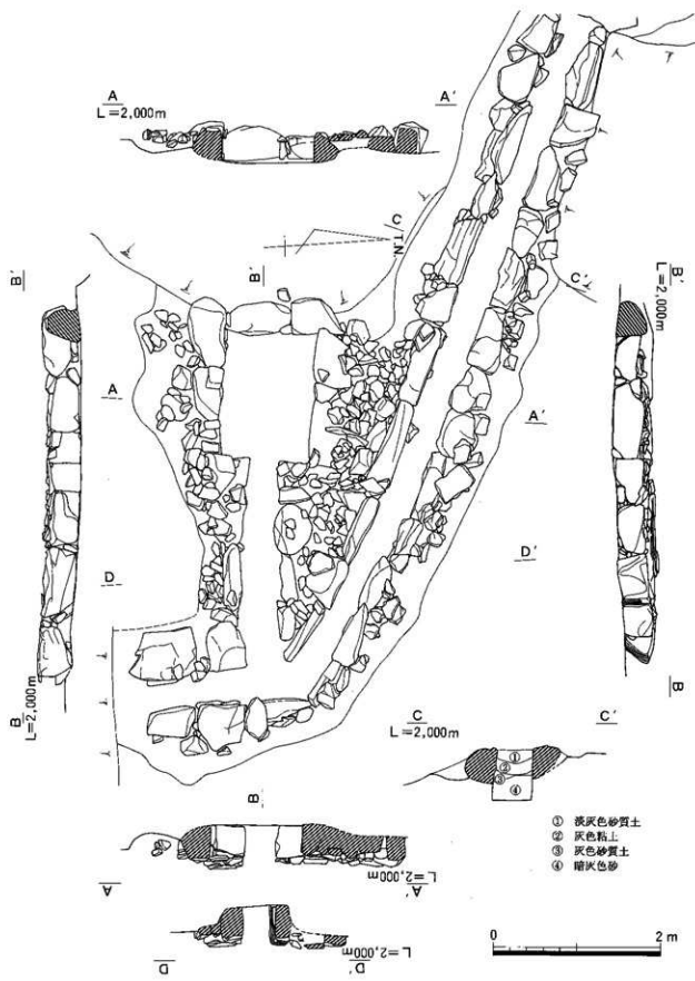
图5 溝01・石室状遺構 平・断面図
