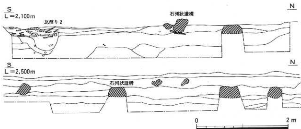
図4 石列状遺構断面図
