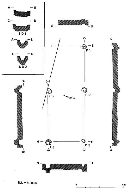
Fig. 9 SB2 · SD1 · SD2 实测图
