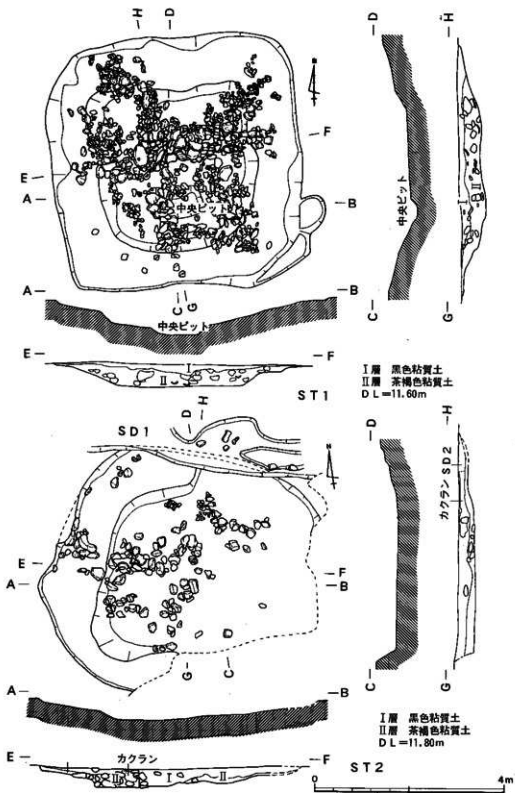
Fig. 7 ST1・ST2 実測図
